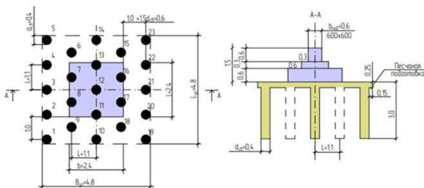
Рисунок 1 – Столбчатые фундаменты: а – на основании, уплотненном песчаными сваями (Источник: составлено авторами)
