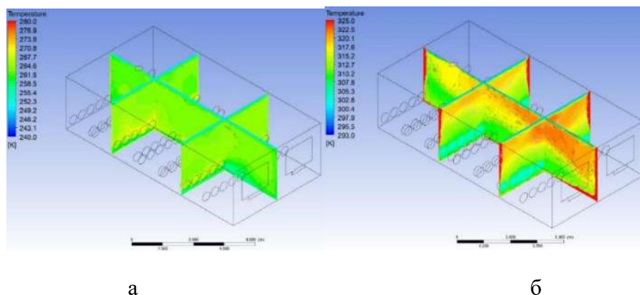
Рисунок 3 – Распределение температуры воздуха в рассматриваемом помещении в холодный период (а) и теплый период (б) (Источник: Составлено автором)
