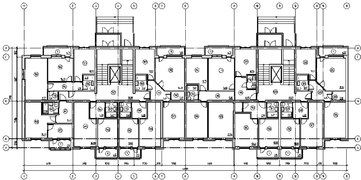
Рисунок 1 – План первого этажа рассматриваемого здания (Источник: Составлено автором)
