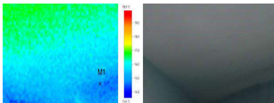
Рисунок 8 – Термограмма покрытия и действительное изображение (Источник: составлено авторами)
