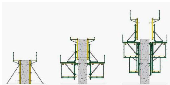
Рисунок 2 – Конструкция самоподъемной опалубки [5]
