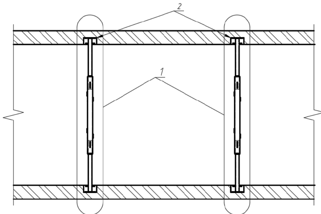
Рисунок 1 – Расположение в плане устройства переменной длины для временного усиления кирпичных стен при демонтаже перекрытий: 1 – устройства переменной длины для временного усиления кирпичных стен при демонтаже перекрытий; 2 – расположенные в кирпичной стене гнезда, которые предназначены для закрепления в них балок перекрытия (Источник: составлено авторами)
