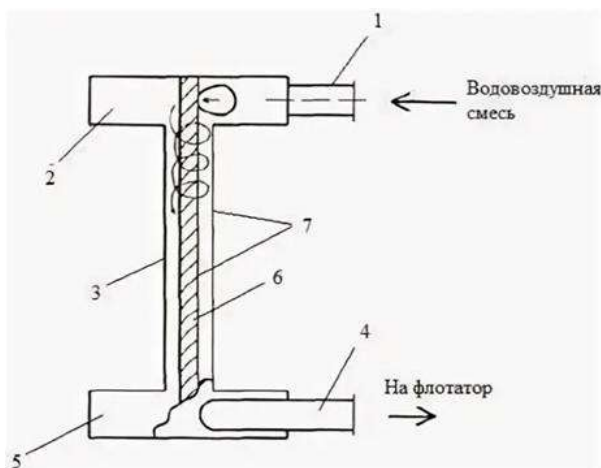
Рисунок 1 – Схема вихревого смесительного устройства (ВСУ) с эмалевым покрытием: 1 – подводящий трубопровод; 2 – входная камера; 3 – ствол (вихревая камера); 4 – центральный стержень; 5 – выходная камера; 6 – выходной трубопровод; 7 – эмалевое покрытие [2]
