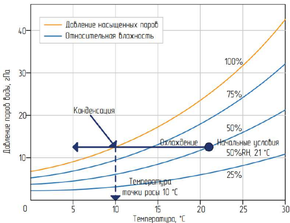
Рисунок 1 – График зависимости температуры точки росы от влажности воздуха в помещении (Источник: Составлено автором)
