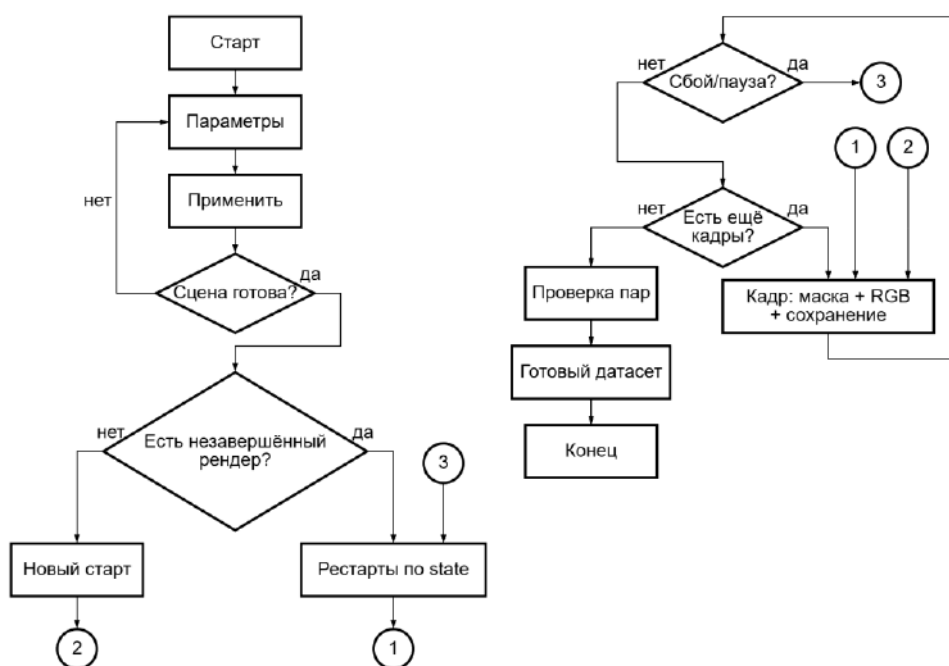
Рисунок 1 – Обобщенная блок-схема алгоритма генерации и рендеринга (Источник: составлено автором Лукьянченко Д.Д.)
