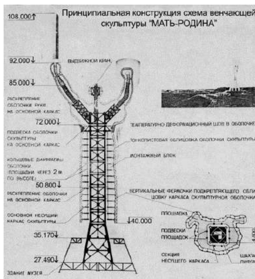
Рисунок 1 – Принципиальная конструктивная схема скульптуры «Родина-мать зовет!» (Источник: [1])
