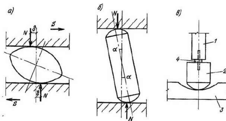
Рисунок 1 – Кинематические опоры, используемые для сейсмоизоляции зданий а – эллипсоиды вращения; б – стойка со сферическими поверхностями торцов; в – опора конструкции Черепинского (1 – колонна; 2 – подколонник; 3 – опорная плита; 4 – центрирующая шайба) (Источник: [4])
