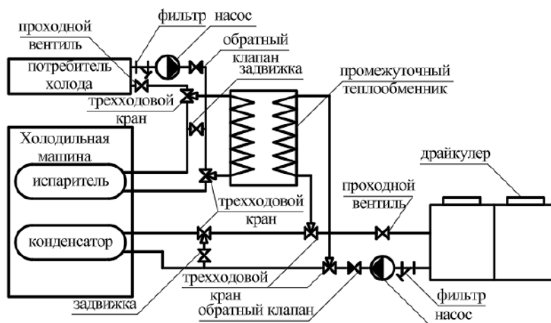
Рисунок 1 – Принципиальная схема системы с технологией фрикулинга
