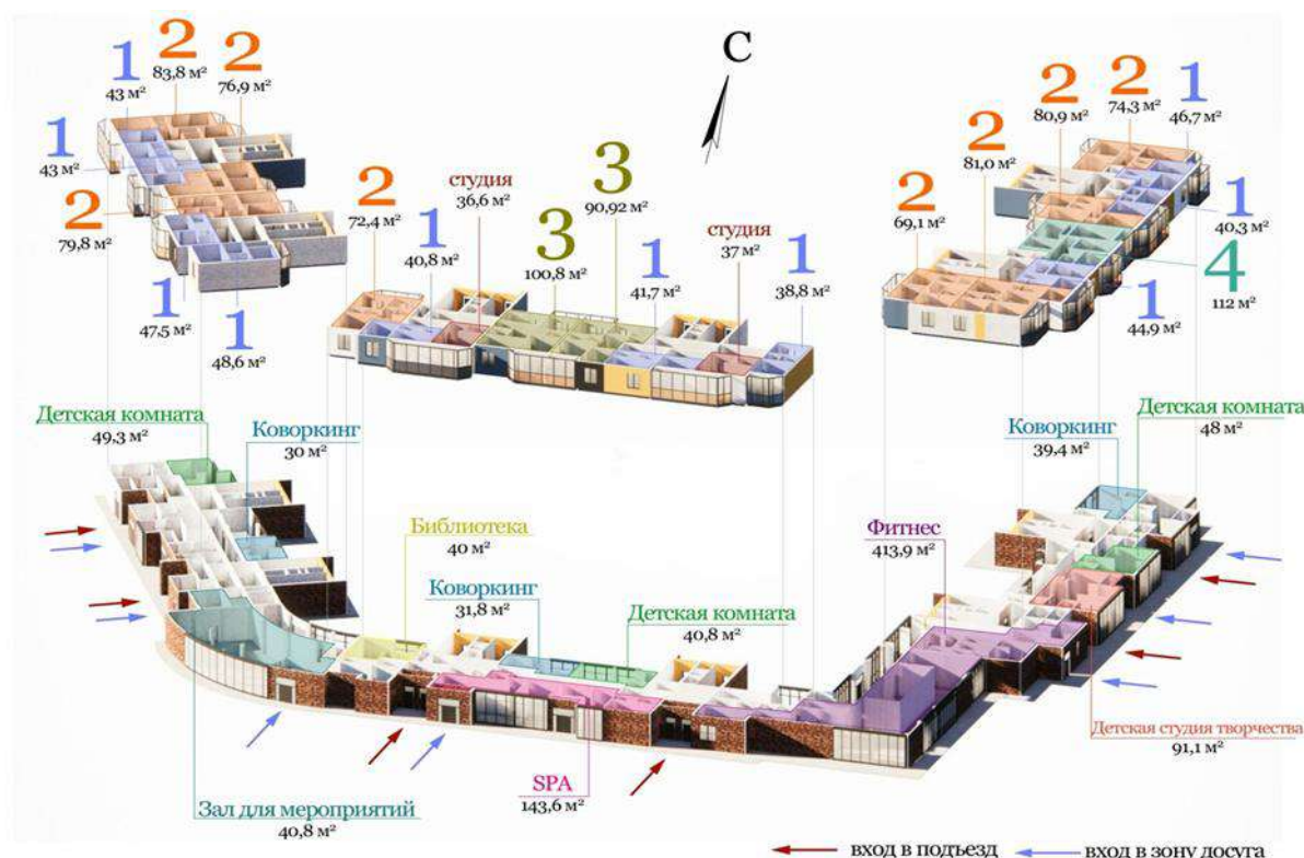
Рисунок 3 – Аксонометрическая схема объемно-планировочных решений досуговых зон и жилого пространства (Источник: Составлено автором)
