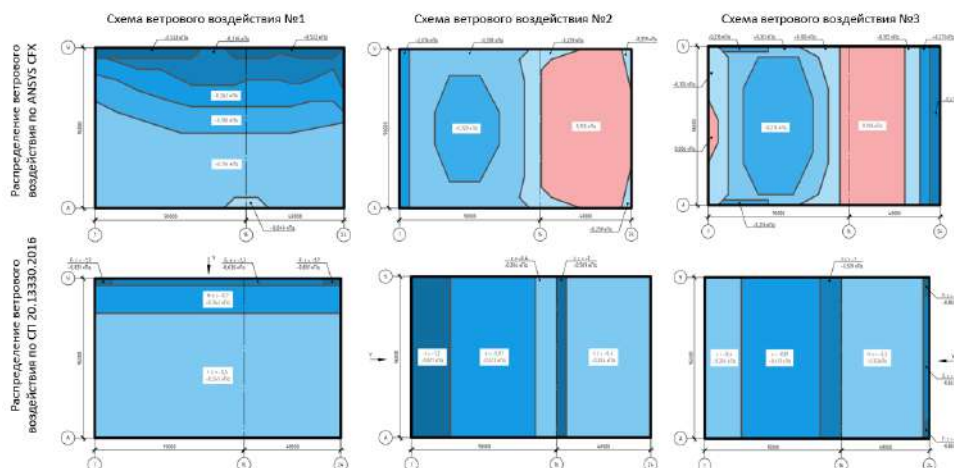
Рисунок 2 – Сравнение полученных результатов расчета в ПБК ANSYS CFX и по СП 20.13330.2016 (Источник: Составлено авторами)
