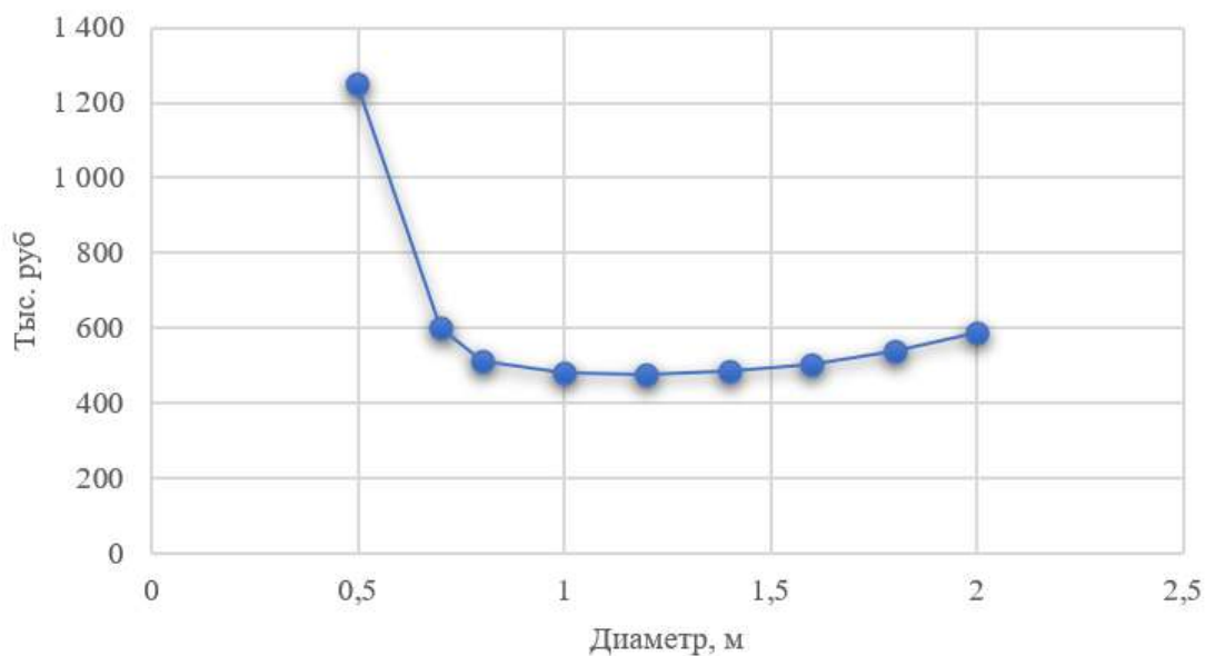
Рисунок 1 – Зависимость суммарных затрат от диаметра вентиляционного канала (Источник: Составлено автором)
