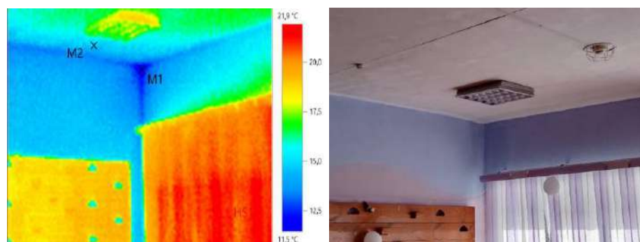
Рисунок 6 – Термограмма стен групповой и действительное изображение (Источник: составлено авторами)
