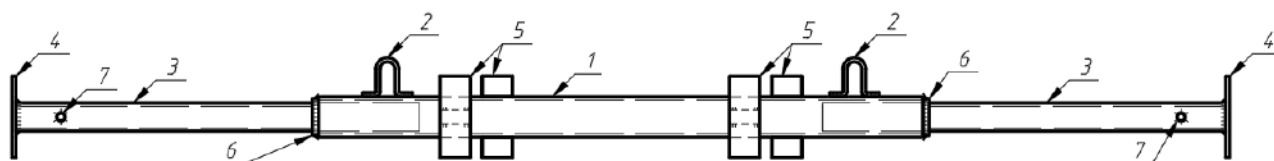
Рисунок 2 – Вид сбоку устройства переменной длины для временного усиления кирпичных стен при демонтаже перекрытий: 1 – неподвижная часть устройства; 2 – монтажные петли; 3 – подвижные части устройства; 4 – стальные упоры; 5 – стальные пластины; 6 – стальные кольца; 7 – стальные ручки (Источник: составлено авторами)
