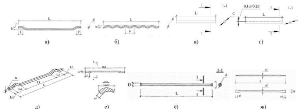
Рисунок 1 – Форма и размеры фибры (Источник: составлено авторами)
