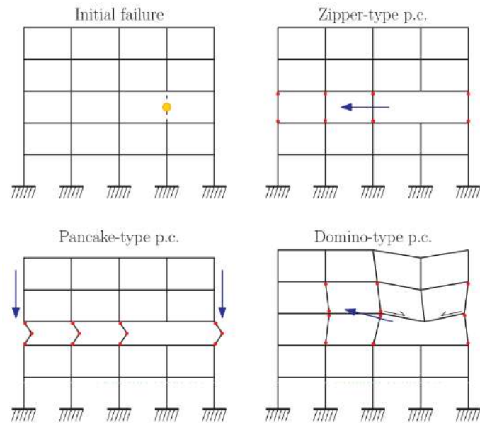
Рисунок 1 – Схемы механизмов прогрессирующего обрушения (Источник: [3])
