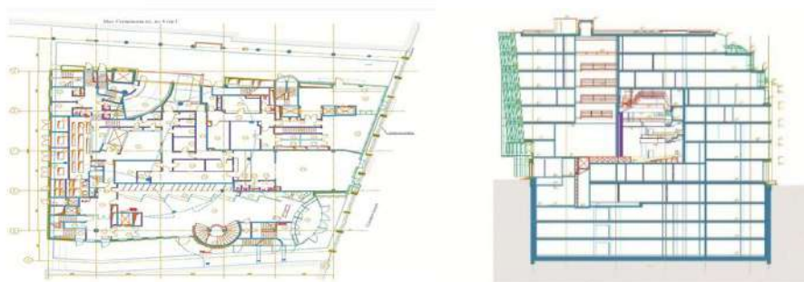
Рисунок 5 – планировка 1 этажа и разрез театрального центра «Вишнёвый сад» в городе Москва
