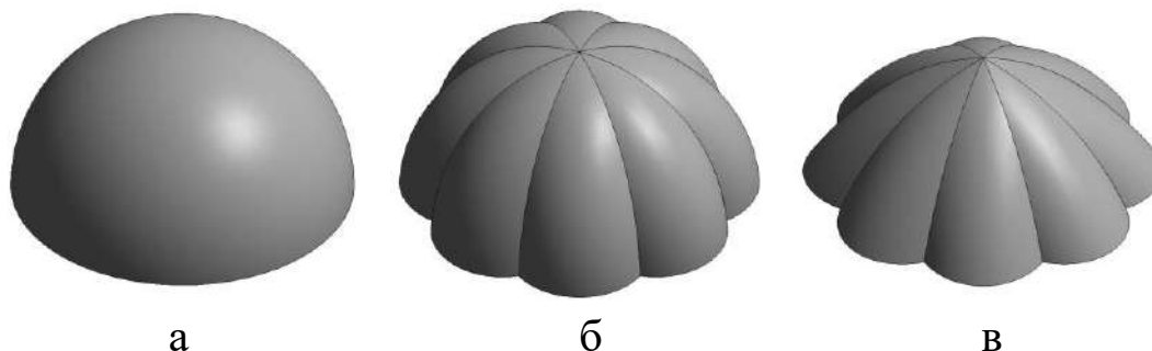
Рисунок 2 – 3D-модель купола: а – гладкий купол, R30, б, в – зонтичная форма с радиусом кривизны R30 и R80 (Источник: составлено авторами)
