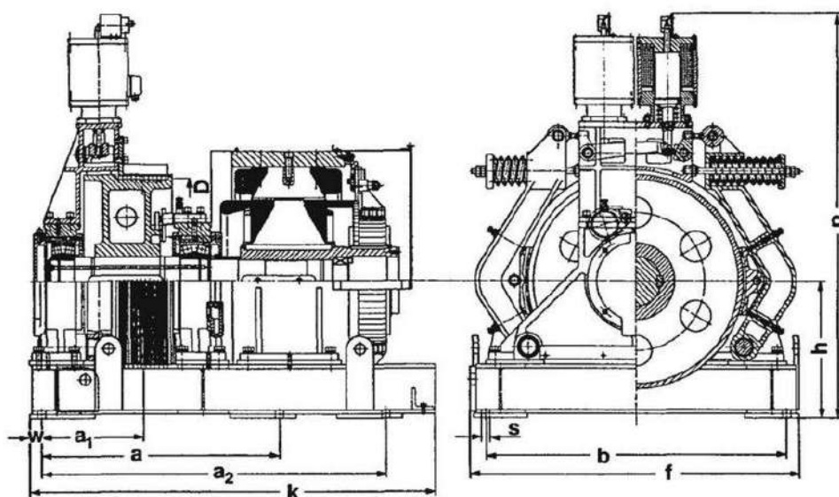
Рисунок 1 – Схема лифтовой безредукторной лебёдки
