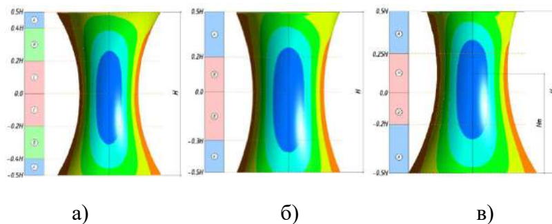
Рисунок 2 – Общий вид картин распределения аэродинамических коэффициентов: а) картина 1; б) картина 2; в) картина 3 пола (Источник: Составлено автором)
