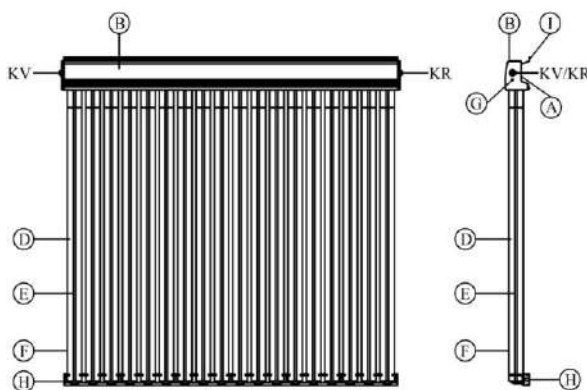
Рисунок 1 – Общий вид солнечного трубчатого коллектора: KV – подающая магистраль коллектора; KR – обратная магистраль коллектора; А – медно-алюминиевый теплообменный блок; В – соединительный корпус коллектора; D – вакуумная стеклянная трубка.; Е – тепловая трубка (Heatpipe); F – поглотитель; I – монтажная шина под стропильный анкер; H – держатель вакуумных трубок; G – проход для датчика температуры [2]
