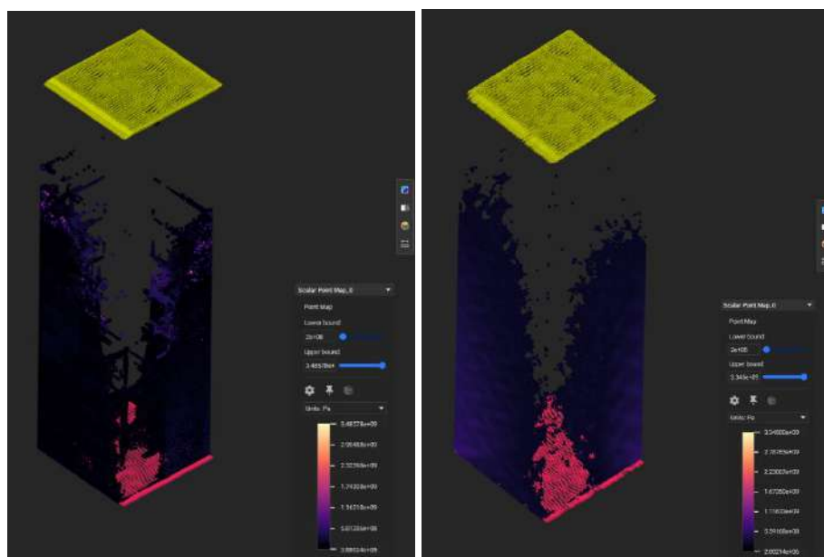
Рисунок 1 – Распределение полей эквивалентных напряжений в ячеистых структурах при однонаправленном нагружении: а) балочная структура; б) структура гироид
