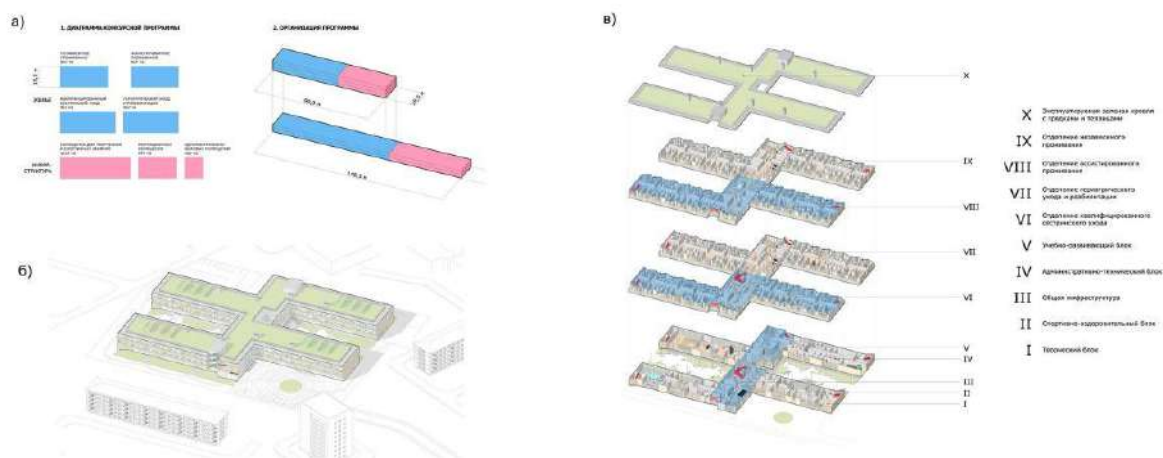
Рисунок 5 – Конкурсный проект геронтологического центра: а) Анализ; б) Модель проекта; в) Функциональная схема [11]
