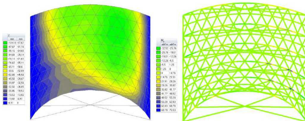
Рисунок 3 – Цветовое отображение вертикальных перемещений и изгибающих моментов при загрузжении – снег на весь пролет (Источник: составлено авторами)
