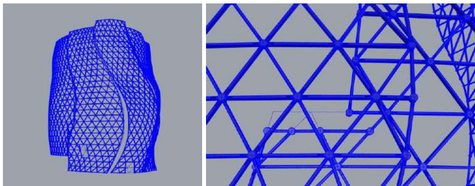
Рисунок 4 – Сетчатая структура здания
