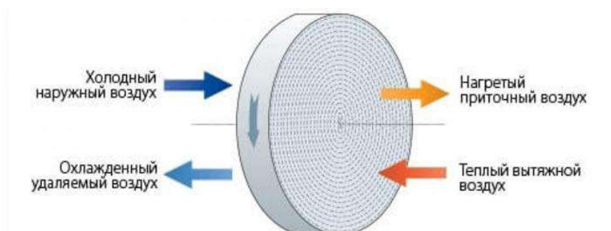
Рисунок 3 – Принципиальная схема работы регенеративного теплообменника [5]
