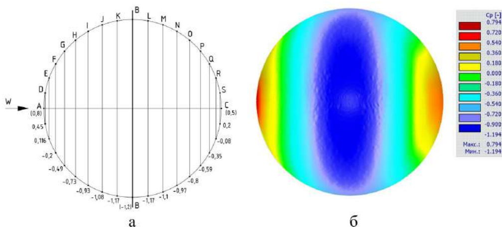
Рисунок 5 – Значения аэродинамических коэффициентов: а – расчетный метод, б – численное моделирование (Источник: составлено авторами)
