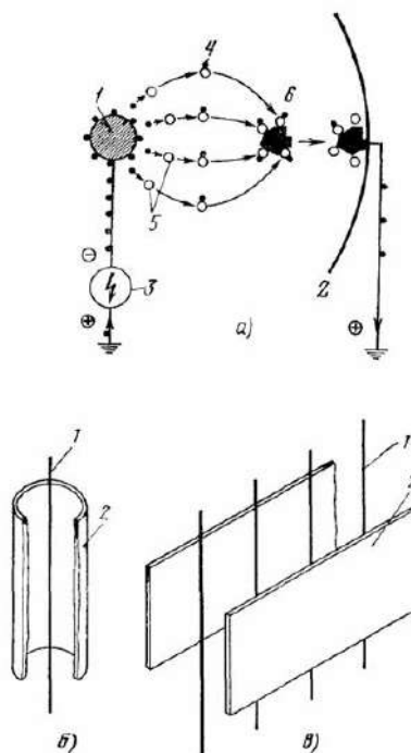
Рисунок 4 – Принципиальная схема работы электрофильтра: а – процесс электрического осаждения частиц; б – электрофильтр с трубчатым электродом; в – электрофильтр с пластинчатыми электродами; 1 – коронирующий электрод; 2 – осадительный электрод; 3 – агрегат электропитания; 4 – электрон; 5 – молекула газа; 6 – осаждаемая частица [1]
