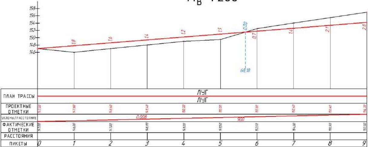
Рисунок 2 – Профиль трассы (Источник: Составлено автором)
