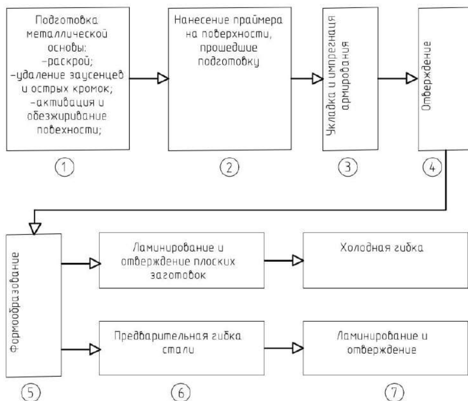
Рисунок 1 – Блок-схема производства углесталеволоконного профиля (Источник: составлено авторами)
