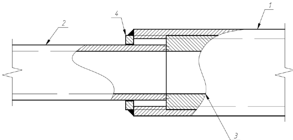
Рисунок 4 – Узел сопряжения подвижной и неподвижной части устройства: 1 – неподвижная часть устройства; 2 – подвижная часть устройства; 3 – стальная втулка; 4 – стальное полукольцо (Источник: составлено авторами)
