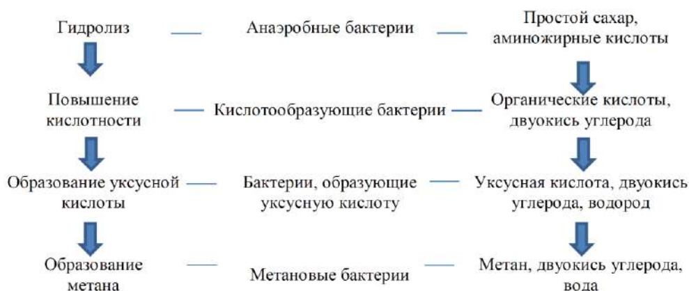
Рисунок 1 – Основные этапы технологии разложения органического субстрата, (составлено авторами)
