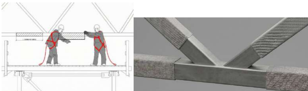
Рисунок 2 – Монтаж огнезащитной сетки на прямолинейных участках конструкции (Источник: Составлено автором)
