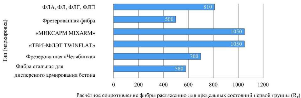
Рисунок 2 – Гистограмма расчётного сопротивления для разных видов фибры (Источник: составлено авторами)
