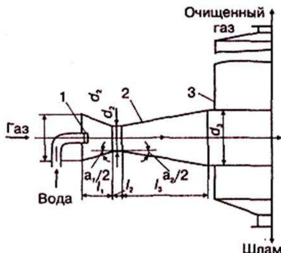
Рисунок 3 – Общий вид и конструкция скруббера Вентури: 1 – форсунки; 2 – сопло Вентури; 3 – каплеуловитель [1]
