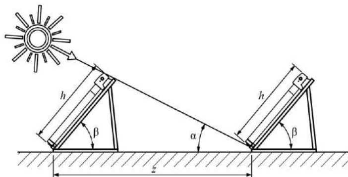
Рисунок 3 – Методика определения расстояния между рядами коллекторов [3]
