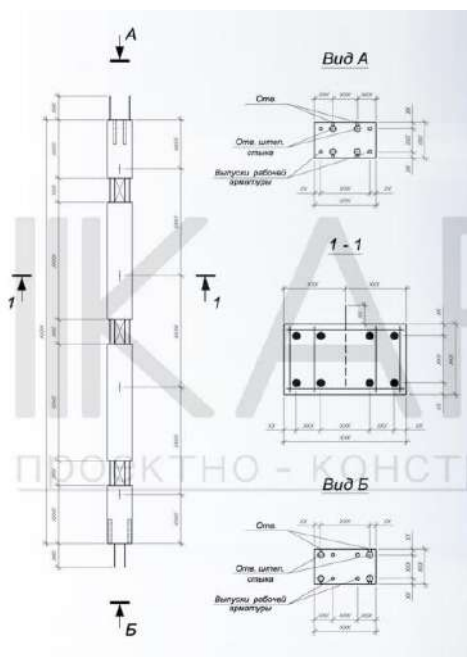
Рисунок 3 – Чертеж колонны системы «Казань XII» адаптированной технологии
