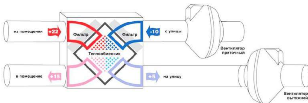
Рисунок 2 – Принципиальная схема устройства пластинчатого рекуператора [5]
