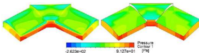
Рисунок 1 – Сравнение результатов компьютерного (слева) и экспериментального физического (справа) моделирования аэродинамического обтекания (Источник: [2])
