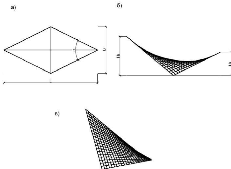
Рисунок 3 – Модель гипара: а – вид сверху; б – вид спереди; в – изометрия (Источник: Составлено автором)
