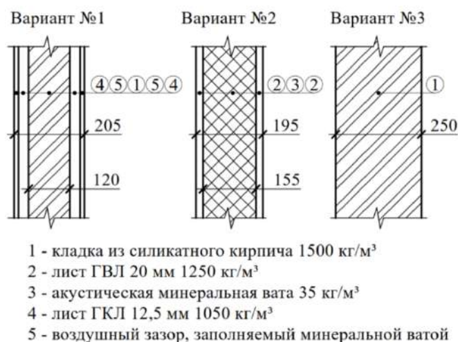
Рисунок 3 – Конструктивное решение ограждений, рассматриваемых в рамках вариантного проектирования замены конструкции №1 (Источник: составлено авторами)
