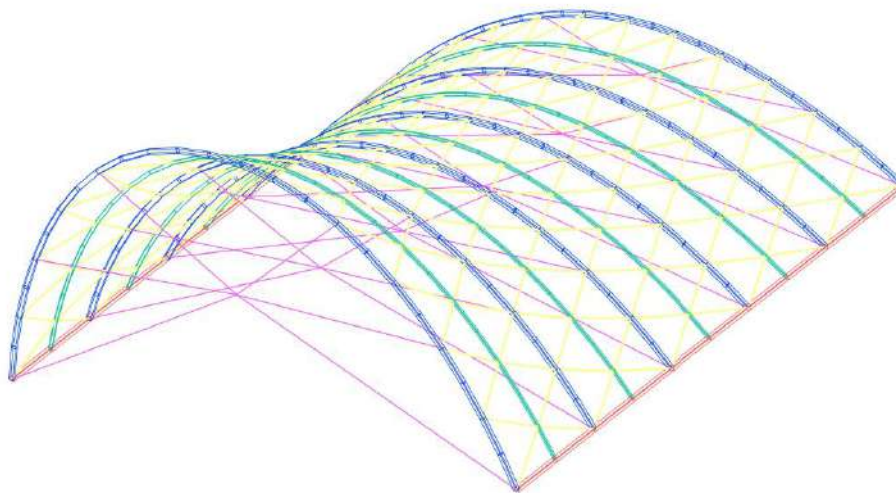
Рисунок 2– Схема покрытия (группы конструктивных элементов выделены разными цветами) (Источник: составлено авторами)
