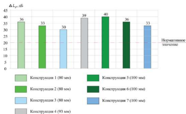
Рисунок 1 – Сравнение значений индексов улучшения изоляции ударного шума за счет различных подложек под стяжку плавающего пола (Источник: составлено авторами)
