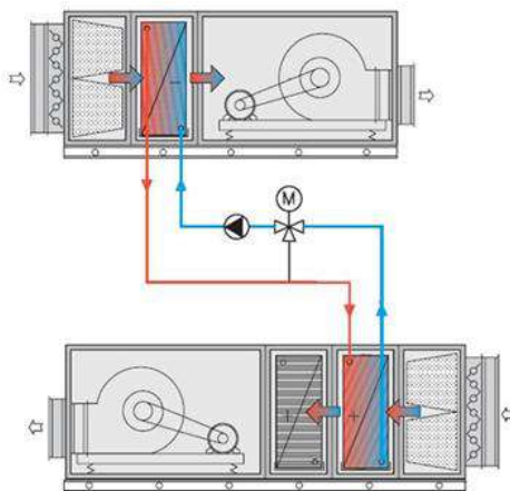
Рисунок 4 – Принципиальная схема работы рекуператора с промежуточным теплоносителем [5]
