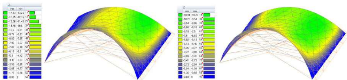
Рисунок 5 – Цветовое отображение вертикальных перемещений на первом и последнем этапе натяжения (Источник: составлено авторами)
