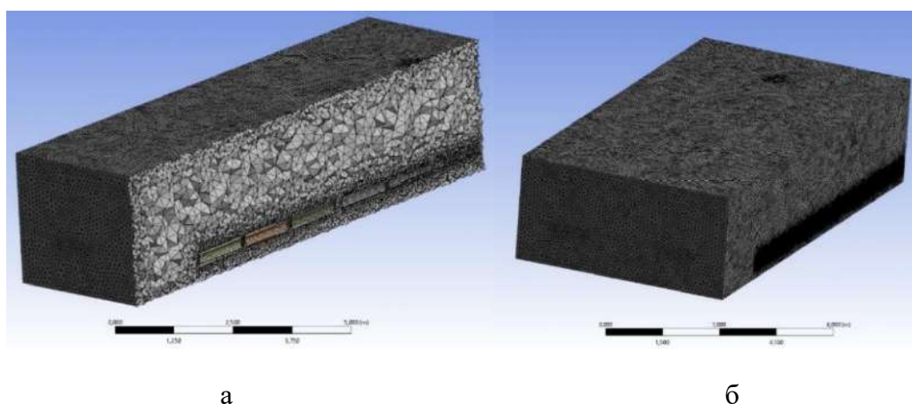
Рисунок 2 – Расчетная сетка помещения (а) и в поперечном сечении (б), сформированная в Ansys Meshing (Источник: Составлено автором)
