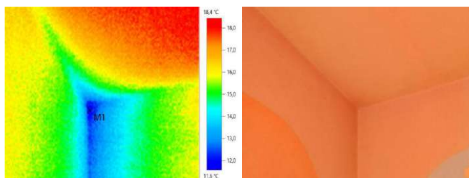
Рисунок 5 – Термограмма стен коридора и действительное изображение (Источник: составлено авторами)
