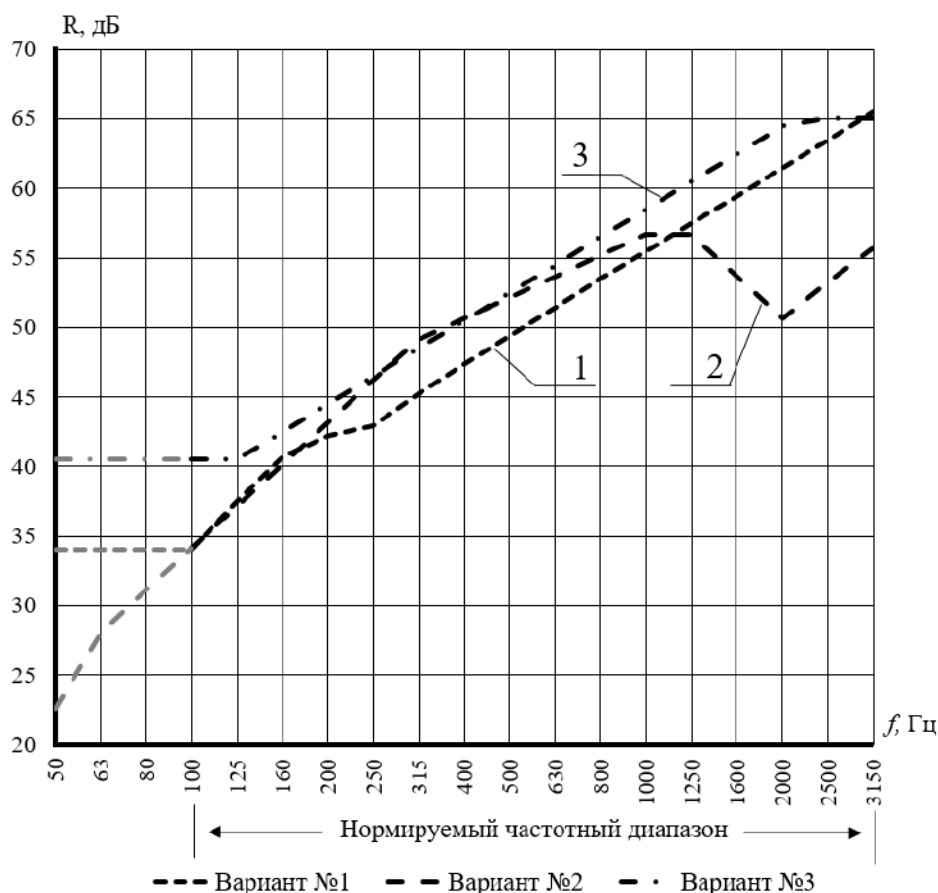
Рисунок 4 – Частотные характеристики звукоизоляции рассматриваемых вариантов конструкций для замены конструкции №2 (Источник: составлено авторами)
