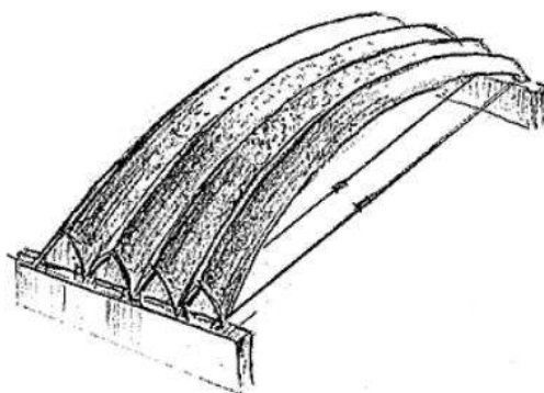
Рисунок 5 – Сводчатые оболочки
