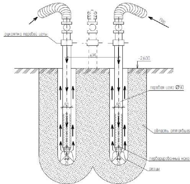
Рисунок 1 – Схема конструкции паровой иглы для оттаивания мерзлых грунтов
