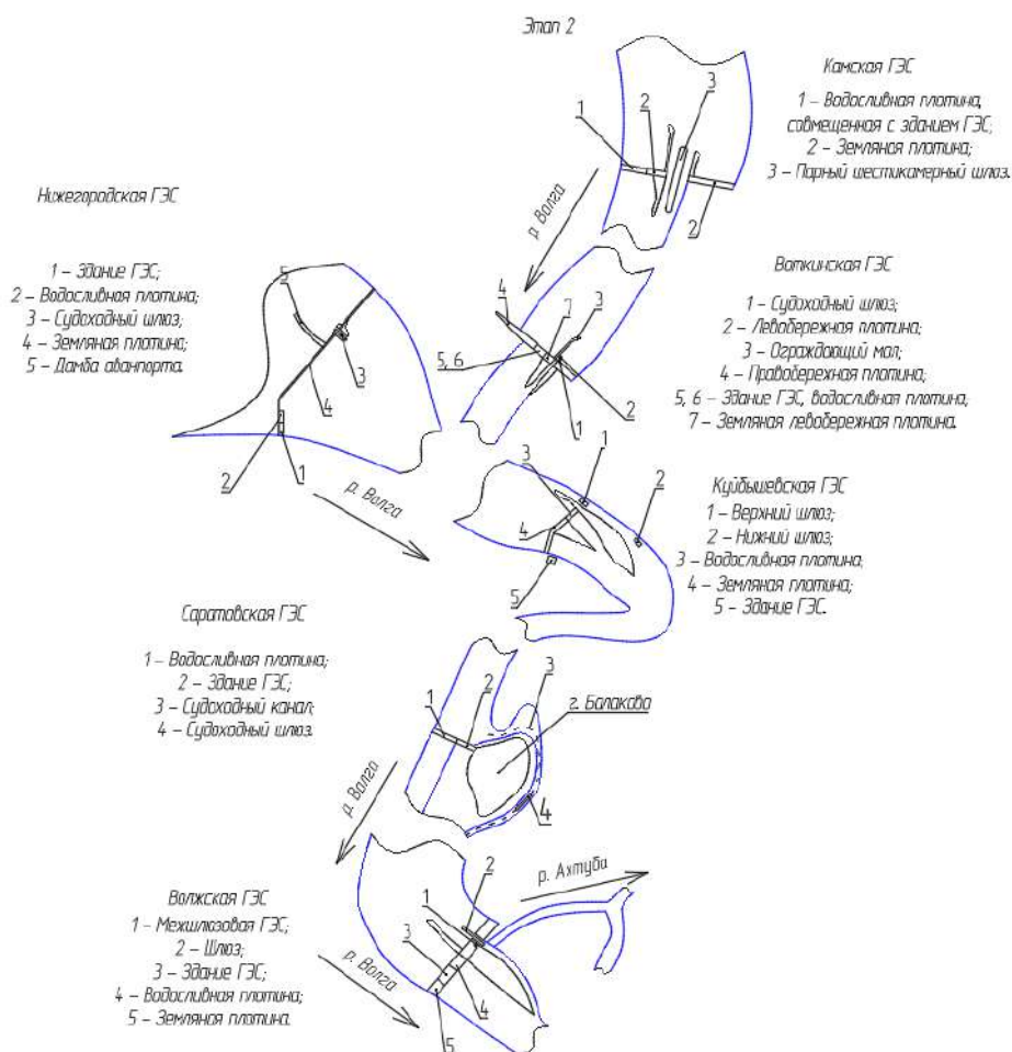
Рисунок 2 – Эволюция компоновок гидроузлов Волжско-Камского каскада – этап 2 (Источник: составлено авторами)
