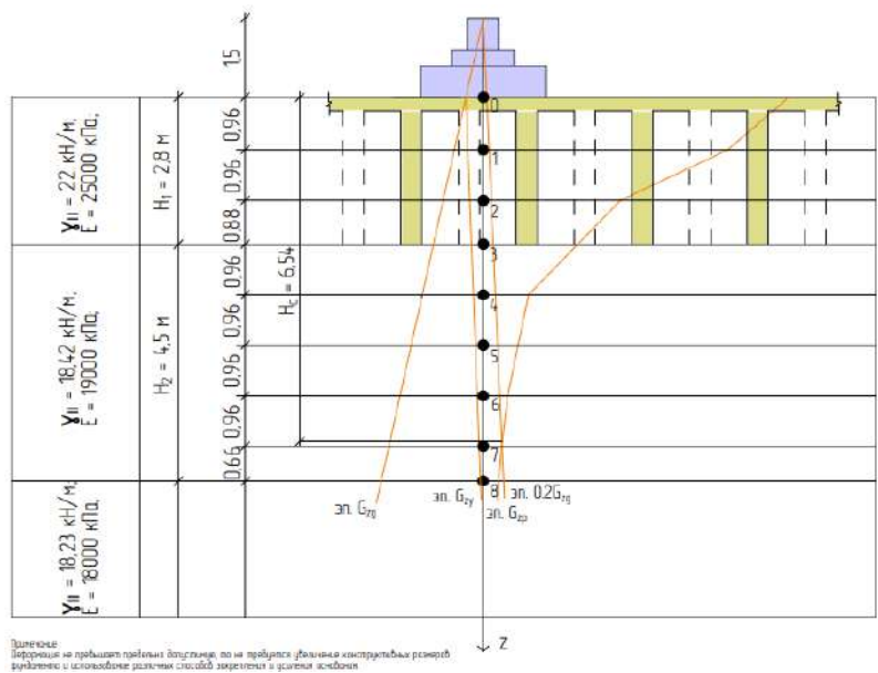
Рисунок 2 – Определение осадки методом послойного суммирования (Источник: составлено авторами)
