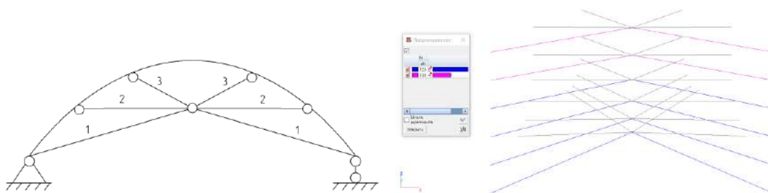
Рисунок 4 – Порядок задания предварительного натяжения канатам. Задание предварительного натяжения нижним затяжкам в ПВК SCAD++ (Источник: составлено авторами)
