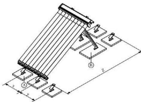
Рисунок 2 – Общий вид смонтированного солнечного трубчатого коллектора: А – передняя опорная пластина; В – задняя опорная пластина; С – монтажная шина под стропильный анкер; x – расстояние между опорами коллектора; y – расстояние между смежными опорами коллекторов; z – расстояние между рядами коллекторов [2]
