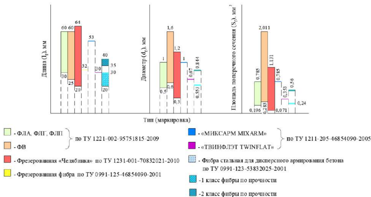
Рисунок 3 – Гистограммы геометрических характеристик для разных видов фибры (Источник: составлено авторами)
