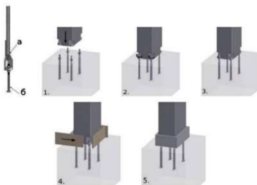
Рисунок 1 – Узловое соединение РЕС компании Reikko и стадии монтажа колонны с применением системы РЕС: а – башмак колонны; б – анкерный болт; 1 – установка колонны на выверенные гайки; 2 – накручивание верхних гаек; 3 – затяжка верхних гаек; 4 – заливка базы колонны безусадочным раствором; 5 – готовое соединение [5]
