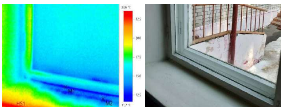
Рисунок 3 – Термограмма оконного заполнения и действительное изображение (Источник: составлено авторами)
