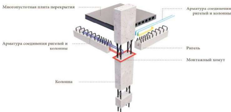
Рисунок 1 – Каркас Сарет
