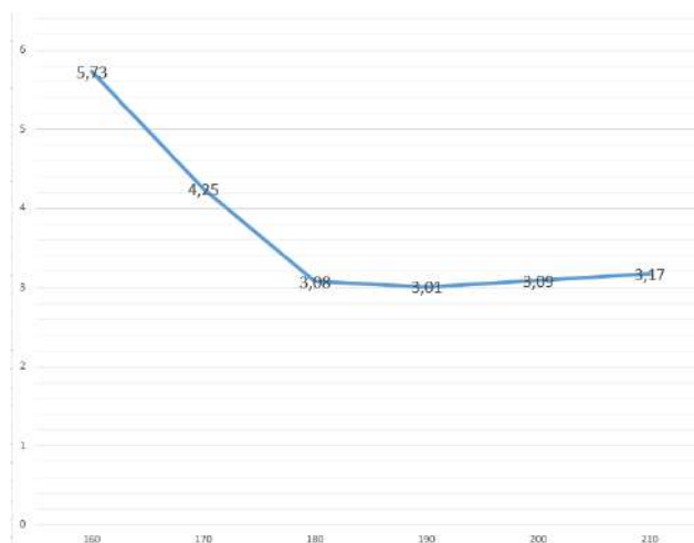
Рисунок 2 – Расход арматуры при загрузении в 1,0 т/м2
