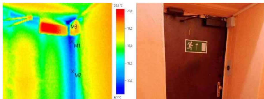
Рисунок 4 – Термограмма входной наружной двери и действительное изображение (Источник: составлено авторами)
