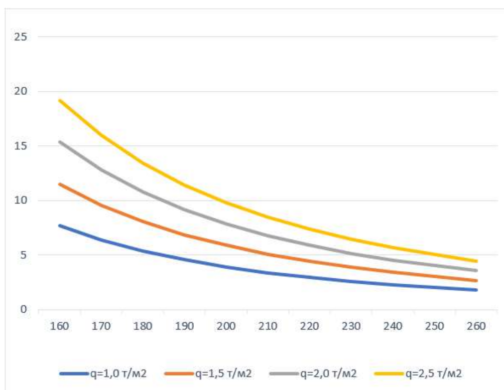
Рисунок 2 – Графики зависимости прогиба в плите перекрытия от толщины при заданной нагрузке
