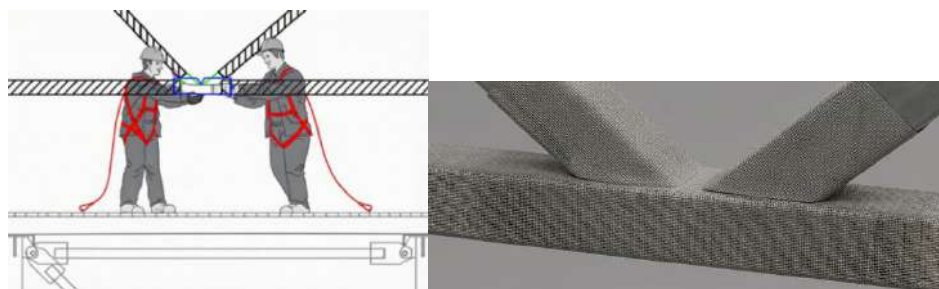
Рисунок 6 – Монтаж огнезащитной сетки на раскосах в местах примыкания к поясам (Источник: Составлено автором)
