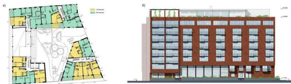
Рисунок 3 – Жилой комплекс «Котисатама»: а) план 1 этажа комплекса; б) внешний вид комплекса [9]
