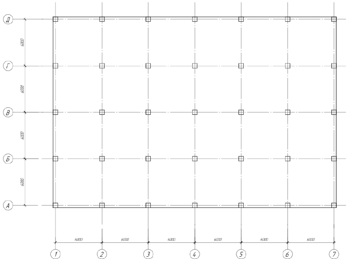
Рисунок 1 – Расчетная схема перекрытия
