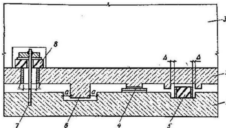
Рисунок 2 – Схема сейсмоизолирующего фундамента со скользящим поясом (Источник [2]). Примечание: 1 – верхняя обвязка фундаментов (стен подвала или технического подполья); 2 – ростверк; 3 – надземная конструкция здания; 4 – скользящая опора; 5 – упругий ограничитель горизонтальных перемещений (демпфер); 6 – жесткий ограничитель горизонтальных перемещений (упор); 7 – ограничитель вертикальных перемещений (вертикальная связь); 8 – вертикальный амортизатор.
