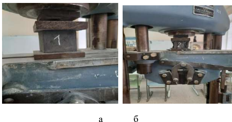
Рисунок 1 – Стадии разрушения образцов из разработанного геополимерного бетона; а – образец перед испытанием, б – разрушенный образец (Источник: составлено авторами)
