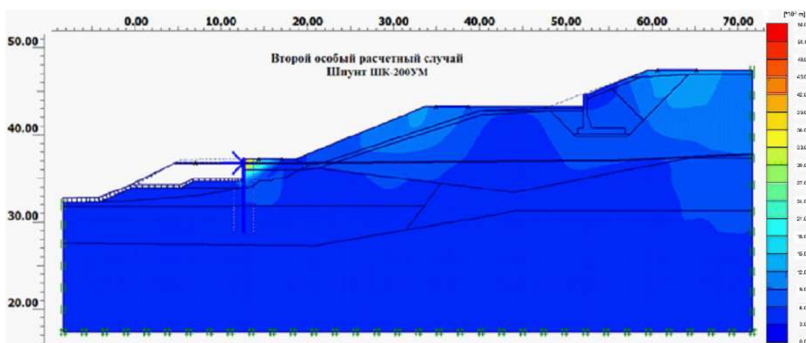
Рисунок 4 – Результаты расчета общей устойчивости берегоукрепления в сечении 1-1. Второй поверочный расчетный случай. Шпунт ШК-200УМ (Источник: Составлено автором)
