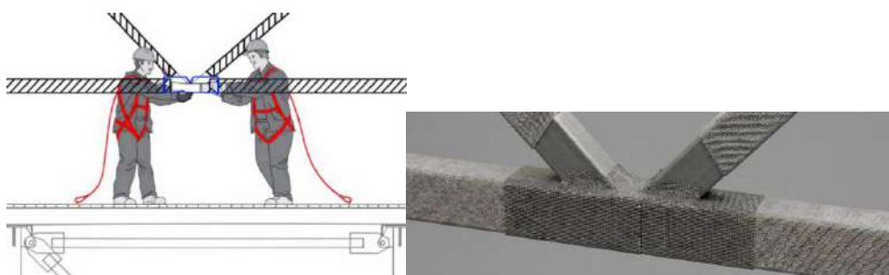
Рисунок 3 – Монтаж огнезащитной сетки в местах примыкания раскосов (Источник: Составлено автором)
