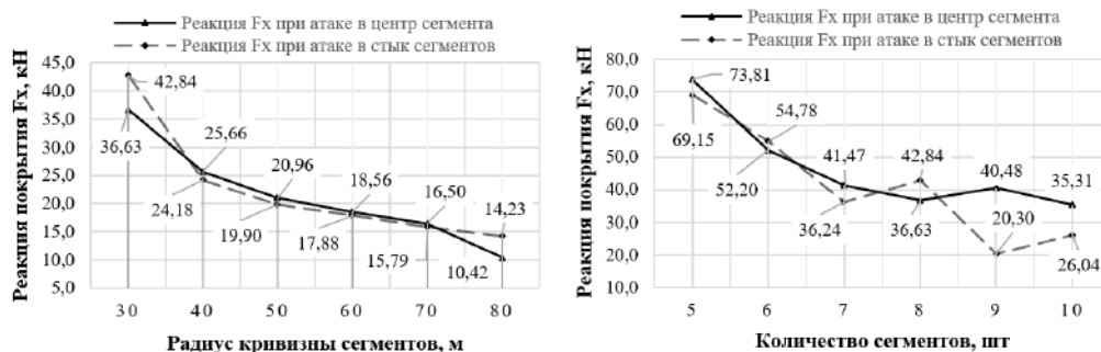
Рисунок 6 – Зависимость реакции покрытия на воздействие ветра от радиуса кривизны сегментов (слева) и количества сегментов (справа) при атаке в центр сегмента и в стык между сегментами (Источник: составлено авторами)
