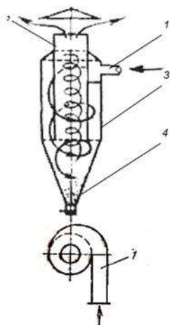
Рисунок 1 – Принципиальная схема циклонного пылеуловителя [1]
