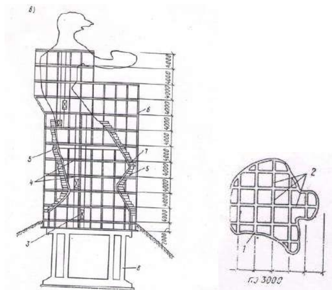
Рисунок 2 – Эскиз монумента «Родина-мать зовёт!» (Источник: [2]); 1 – наружная железобетонная оболочка, 2 – система перекрестных железобетонных стен, 3 – подъемник, 4 – железобетонные перекрытия, 5 – сборные лекала внешней опалубки, 6 – регулярный стальной каркас для возведения монумента, 7 – гипсобетонное заполнение внешней опалубки, 8 – фундамент.
