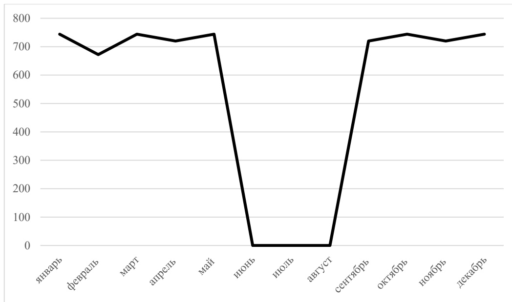
Рисунок 1 – График часов использования технологии Free Cooling относительно месяца
