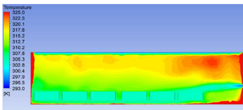
Рисунок 5 – Распределение температуры воздуха в поперечном сечении рассматриваемого помещения в теплый период (Источник: Составлено автором)
