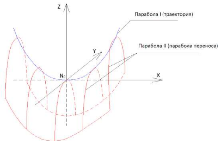
Рисунок 1 – Формообразующие параболического гиперboloида [2]
