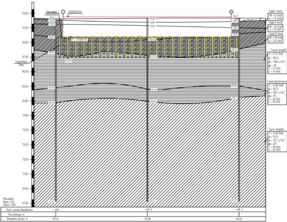
Рисунок 3 – Инженерно-геологический разрез с грунтовыми сваями (Источник: составлено авторами)
