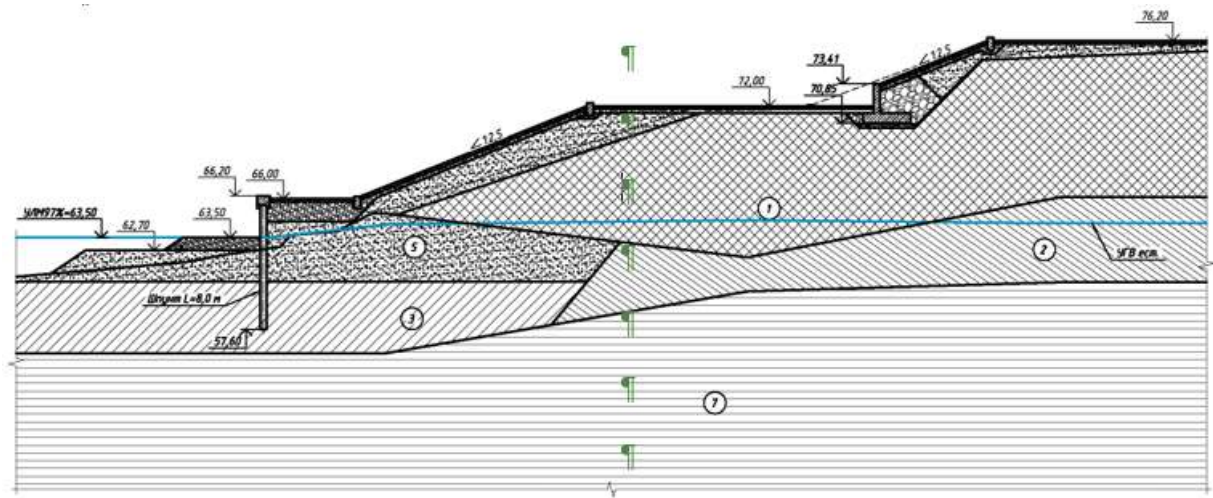
Рисунок 1 – Схема к расчету в сечении 1-1 (Источник: Составлено автором)
