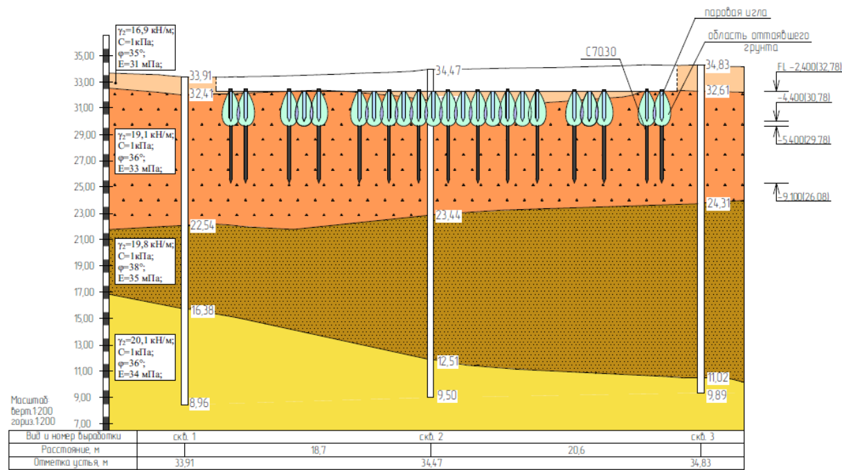
Рисунок 2 – Схема расположения паровых игл и зон оттаивания в грунте на примере проектирования объекта в г. Архангельске
