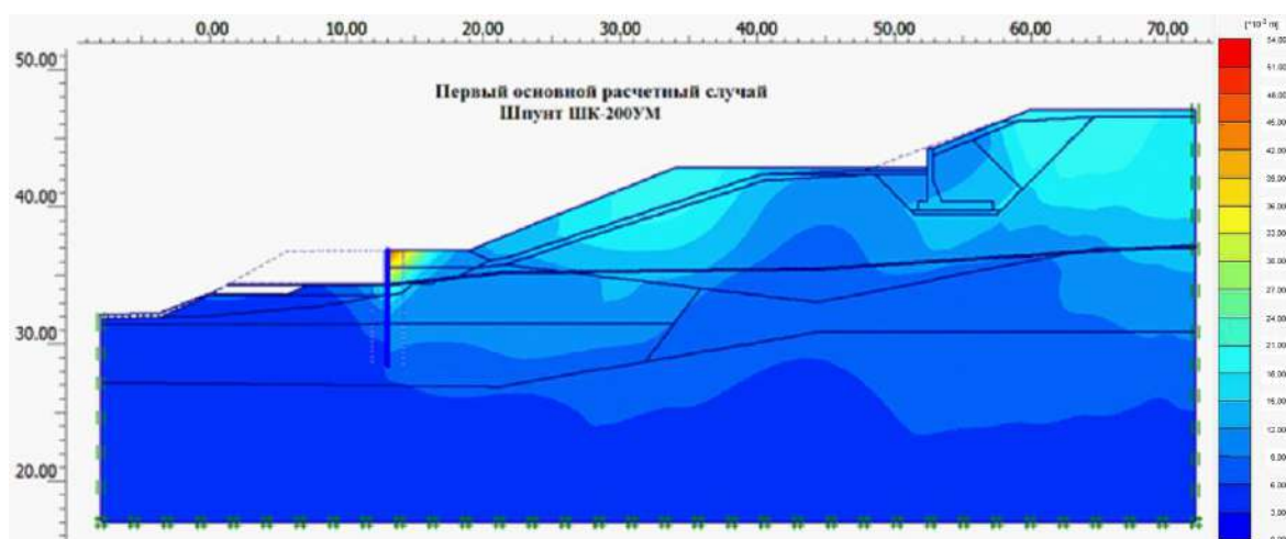
Рисунок 3 – Результаты расчета общей устойчивости берегоукрепления в сечении 1-1. Первый основной расчетный случай. Шпунт ШК-200УМ (Источник: Составлено автором)
