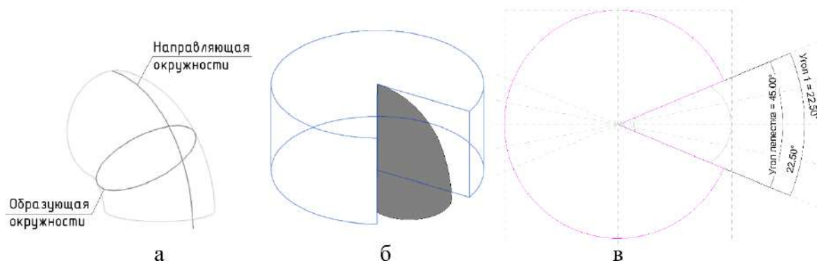
Рисунок 1 – Модель сегмента покрытия: а – схематичный вид, б – фрагмент в усеченном виде, в – задание параметров (Источник: составлено авторами)
