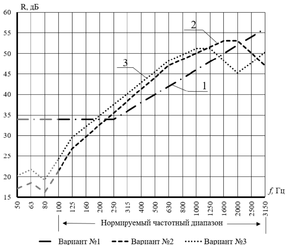
Рисунок 2 – Частотные характеристики звукоизоляции рассматриваемых вариантов конструкций для замены конструкции №1 (Источник: составлено авторами)
