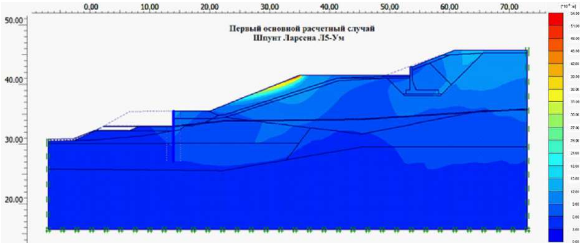
Рисунок 2 – Результаты расчета общей устойчивости берегоукрепления в сечении 1-1. Первый основной расчетный случай. Шпунт Ларсена Л5-УМ (Источник: Составлено автором)
