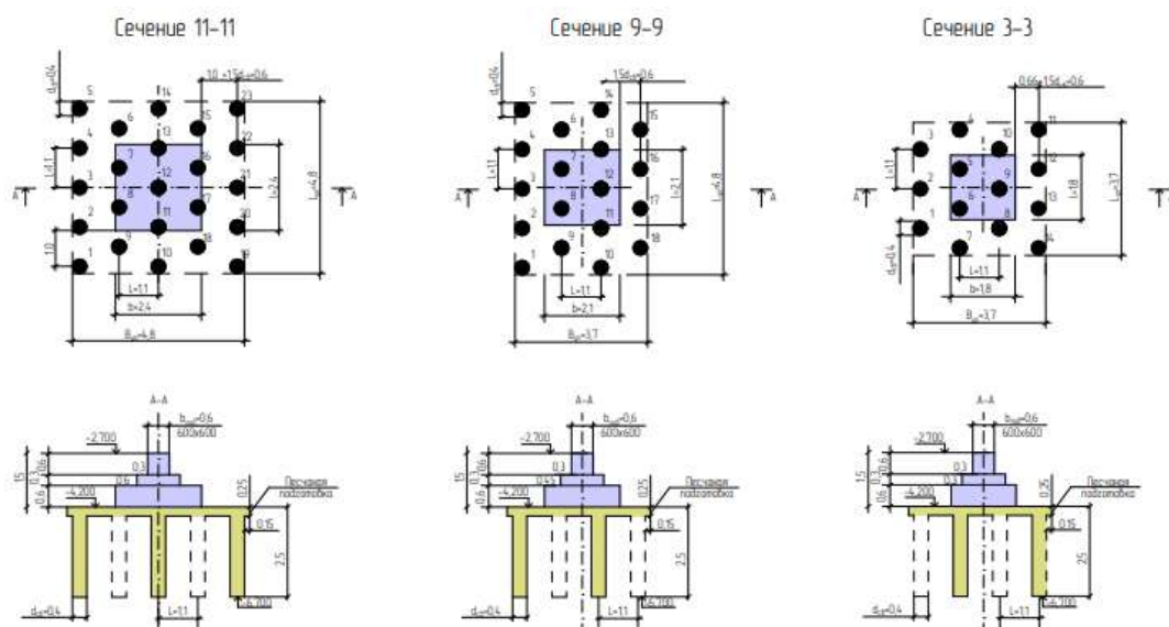
Рисунок 4 – Вариативность сечений (Источник: составлено авторами)
