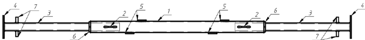
Рисунок 3 – Вид сверху устройства переменной длины для временного усиления кирпичных стен при демонтаже перекрытий: 1 – неподвижная часть устройства; 2 – монтажные петли; 3 – подвижные части устройства; 4 – стальные упоры; 5 – стальные пластины; 6 – стальные кольца; 7 – стальные ручки (Источник: составлено авторами)
