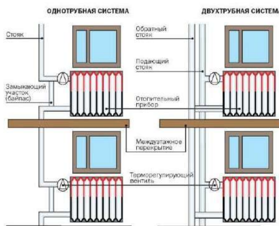
Рисунок 2 – Однотрубная (слева) и двухтрубная система отопления МЖД (справа) (Источник: [3])
