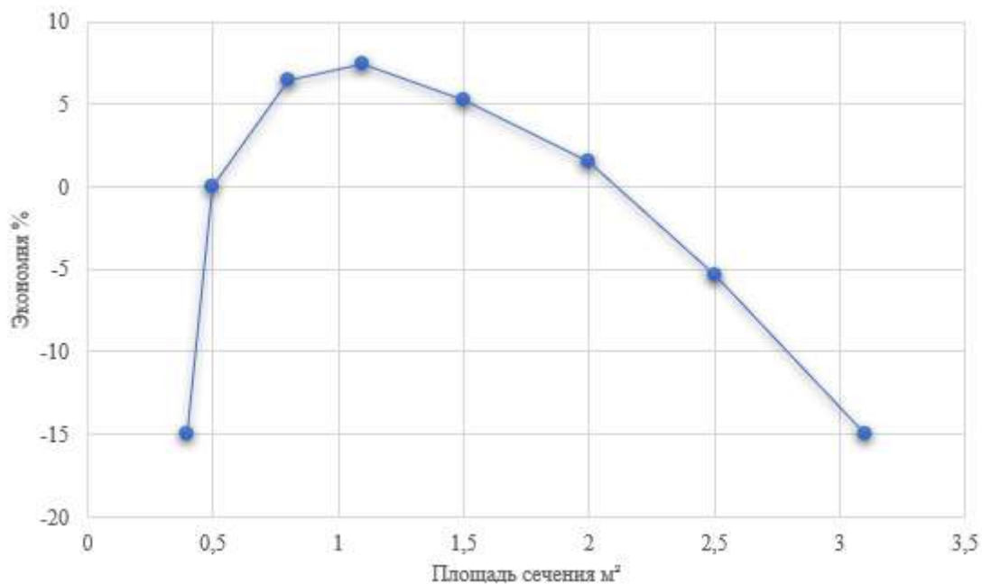
Рисунок 2 – Диаграмма относительной экономии от площади сечения (Источник: Составлено автором)
