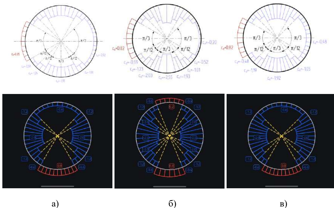
Рисунок 3 – Картинки распределения аэродинамических коэффициентов по расчету сверху – в ПК Ansys CFX; снизу – в автоматизированной системе: а) на отм. +9,900 ; б) на отм. +80,100 ; в) на отм. +150,300 пола (Источник: Составлено автором)
