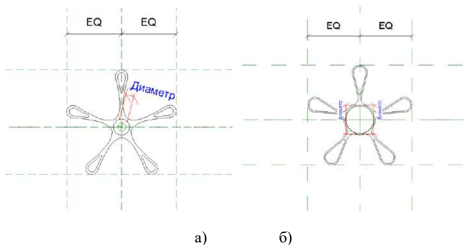
Рисунок 1 – Общий вид параметрических семейств водяных инфракрасных излучателей (Flower 125 (а) и Flower 225 (б)) в среде Autodesk Revit (Источник: Составлено автором)
