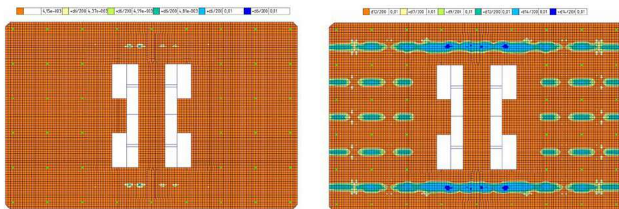
Рисунок 2 – Сравнение изополей армирования; слева – плита с предварительным напряжением, справа – классическая плита (Источник: составлено авторами)
