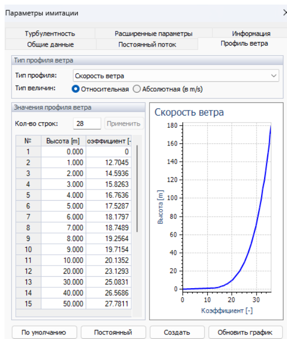
Рисунок 4 – Параметр набегающего потока (Источник: составлено авторами)
