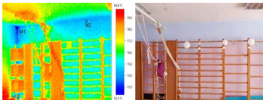
Рисунок 7 – Термограмма стен спортзала и действительное изображение (Источник: составлено авторами)
