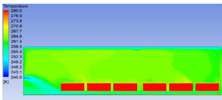
Рисунок 4 – Распределение температуры воздуха в поперечном сечении рассматриваемого помещения в холодный период (Источник: Составлено автором)
