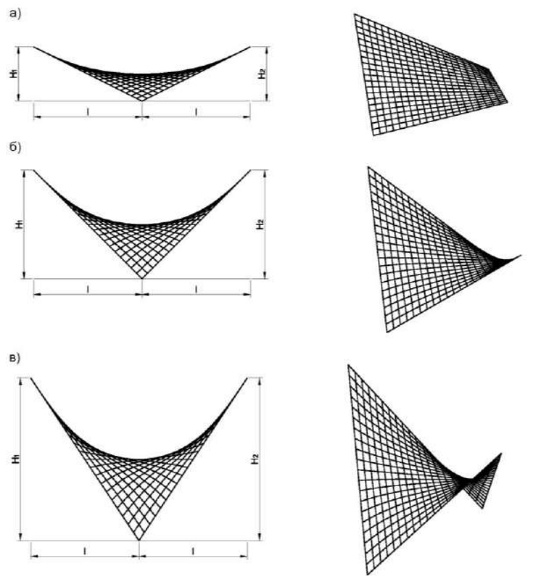
Рисунок 5 – Модели в зависимости от параметров H1 и H2 : а – модель при H1=H2<1 ; б – модель при H1=H2=1 ; в – модель при H1=H2>1 (Источник: Составлено автором)
