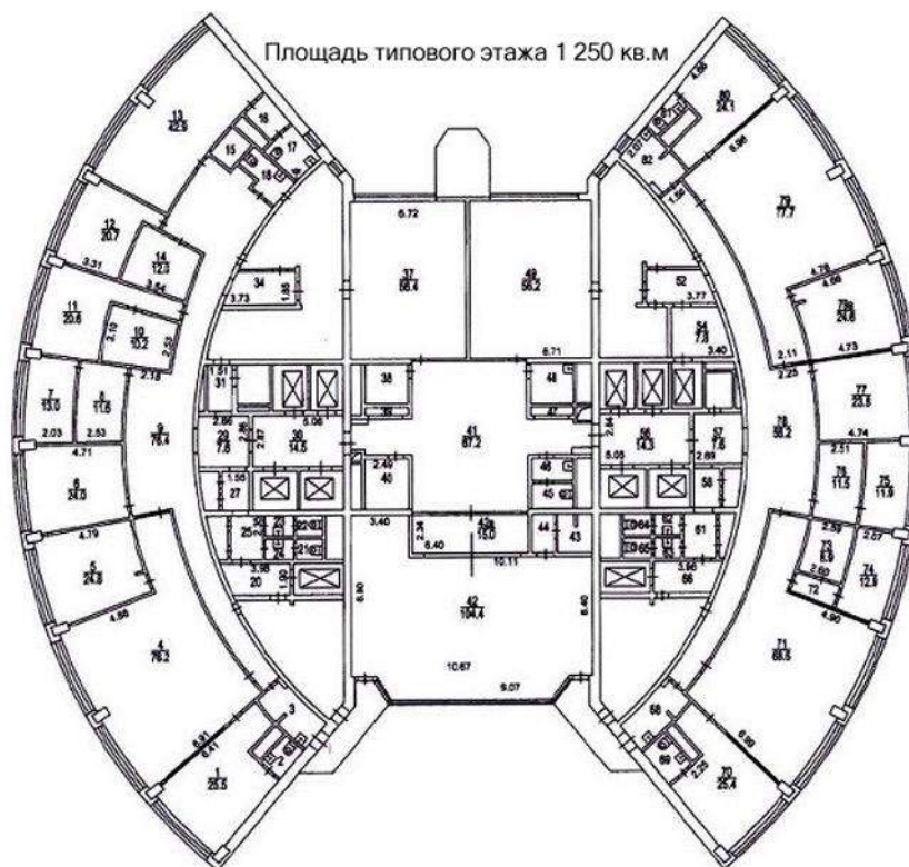
Рисунок 2 – Схема расположения лифтов в «Башня 2000»
