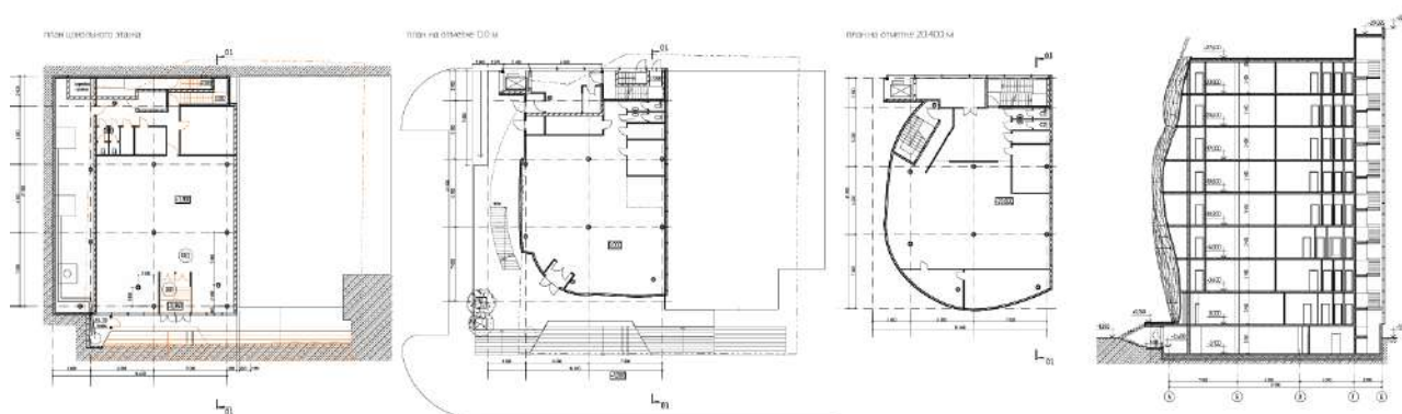
Рисунок 2 – План цокольного этажа, план на отм. 0.000, план на отм. +20.400 и разрез 1-1
