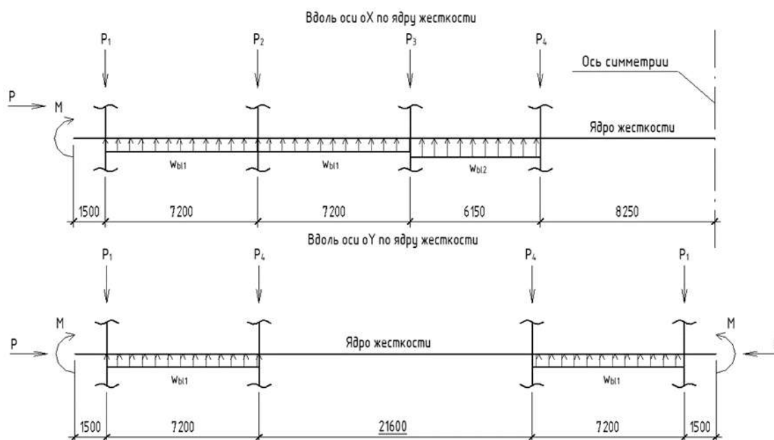
Рисунок 1 – Расчетная схема по идеализированной модели Лина (Источник: [2], [4])
