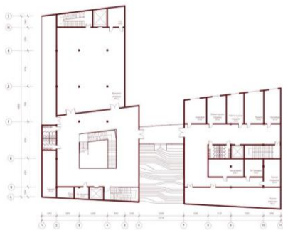
План 2 этажа M 1:200
