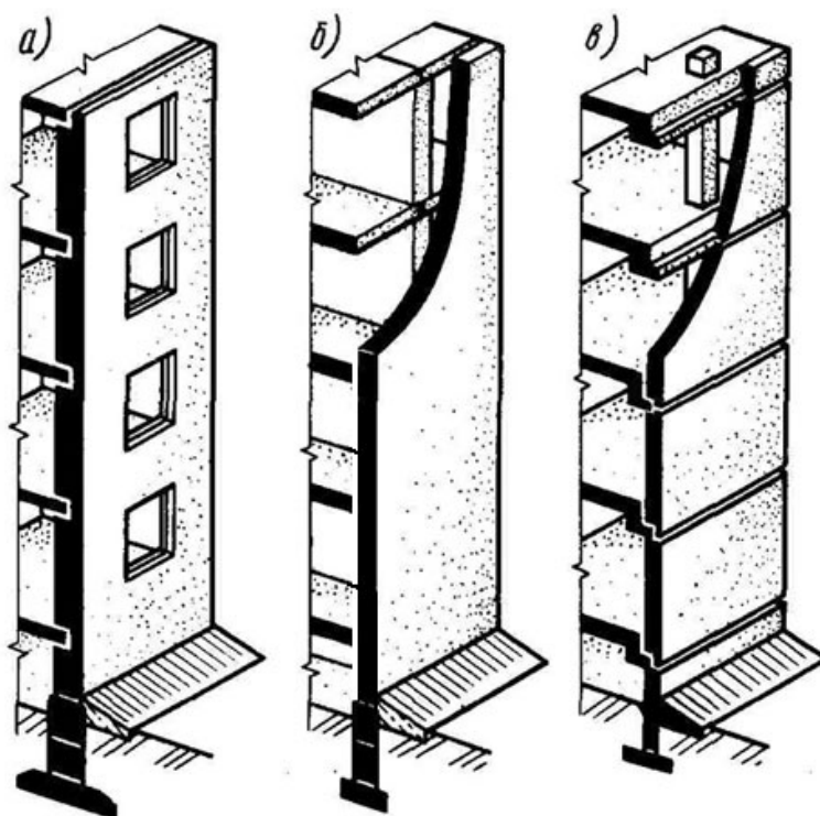
а) несущие; б) самонесущие; в) ненесущие с опиранием на перекрытие
