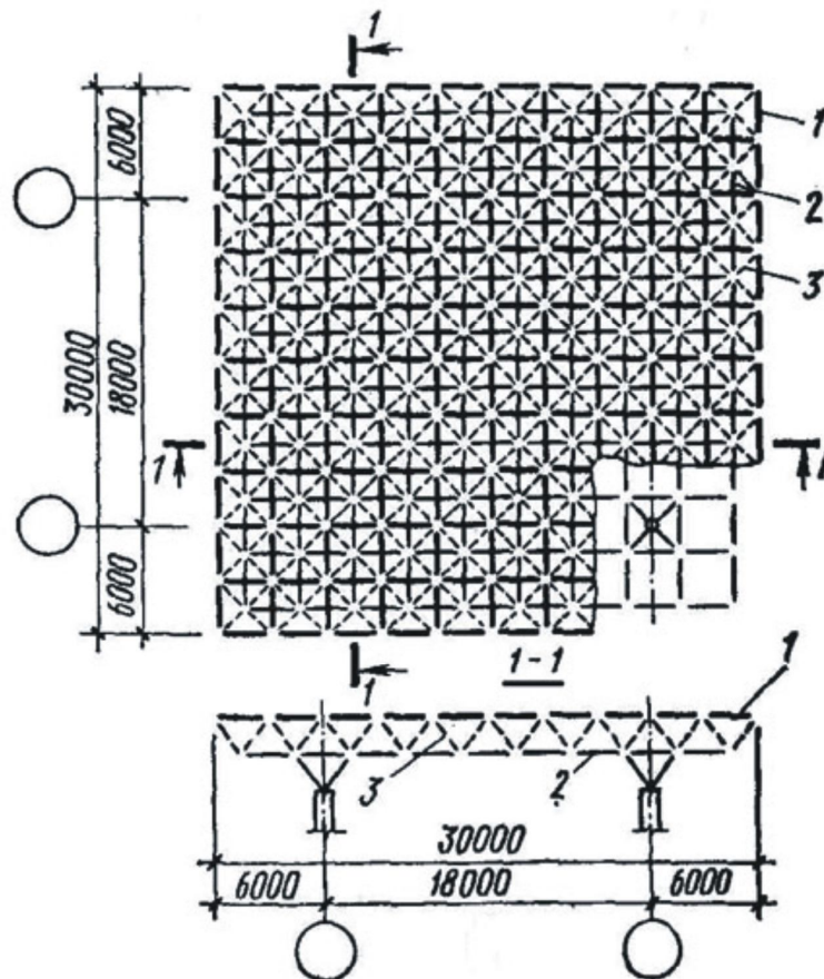
Рис. 21. Перекрёстные системы покрытия
