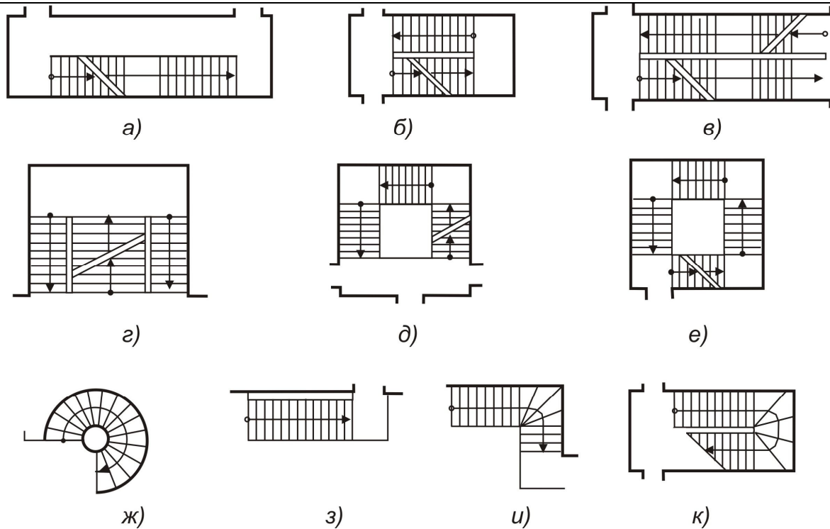
Рис. 7. Типы лестниц
