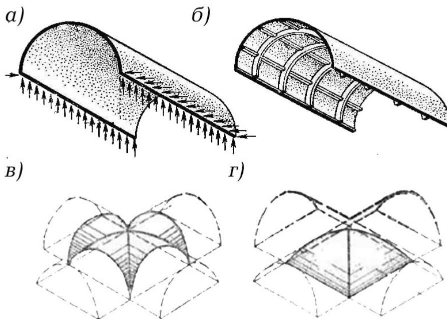
Рис. 22. Своды
