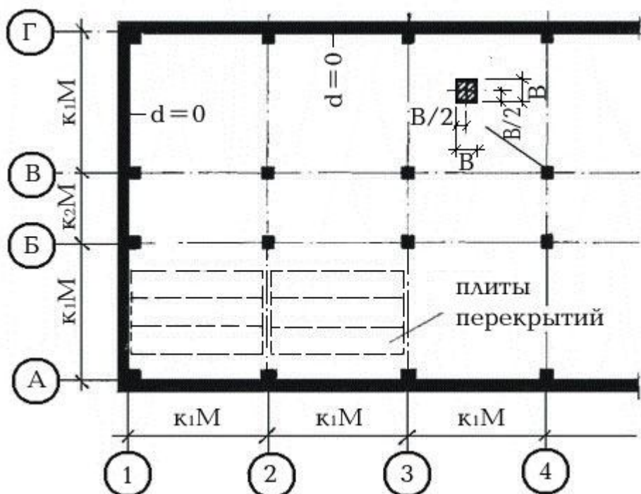
Рис. 5. Привязка к координационным осям колонн и наружных ограждающих конструкций в каркасном здании с навесными или самонесущими стенами
