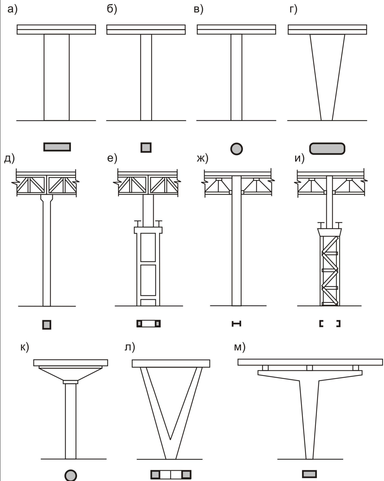
Рис. 19. Формы вертикальных элементов стоечно-балочной конструктивной системы
