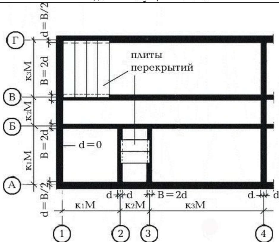
Рис. 4. Привязка к координационным осям конструкций в здании несущими стенами
