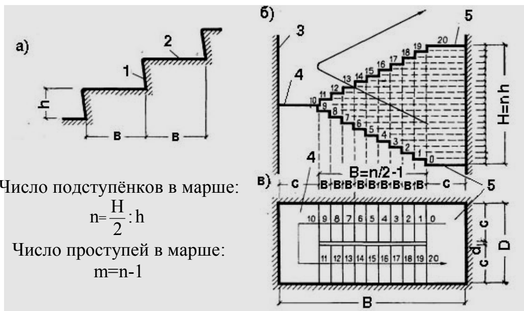
Рис. 8. Геометрическое построение лестницы:
