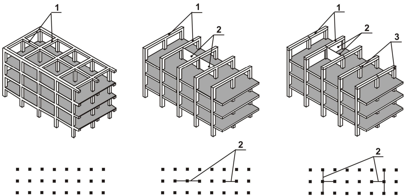
Рис. 16. Виды каркасов
