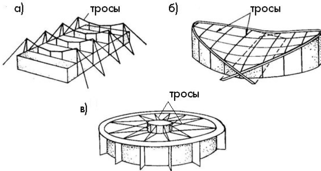
Рис.26. Висячие покрытия
