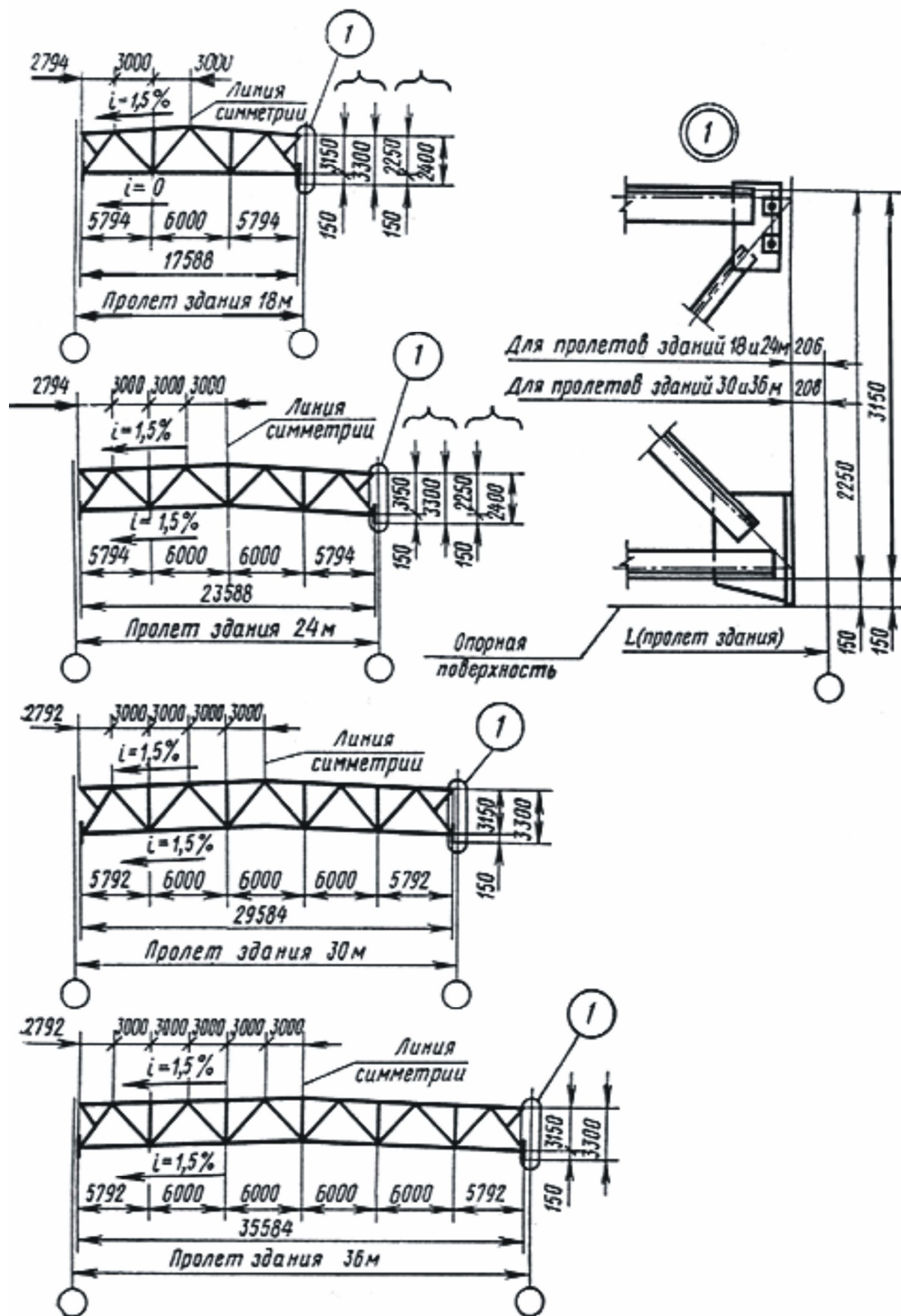
Рис.18.3. Металлические фермы (ГОСТ 23119-78)
