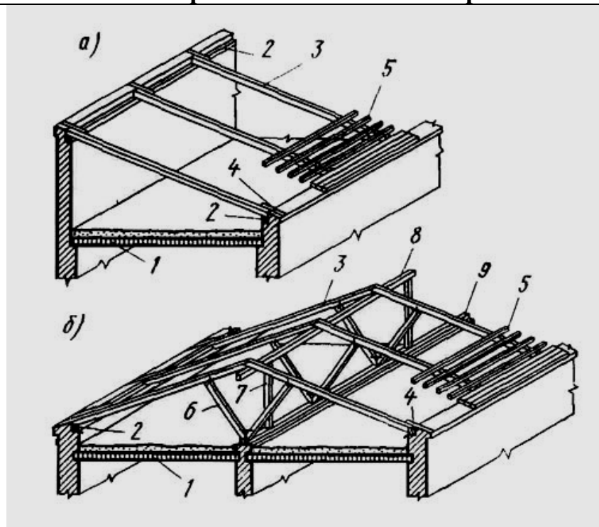
а) односкатная; б) двухскатная; 1 - чердачное перекрытие; 2 - мауэрлат; 3 - стропильные ноги; 4 - кобылка; 5 - обрешётка; 6 - подкос; 7 - стойка; 8 - коньковый прогон; 9 - лежень
