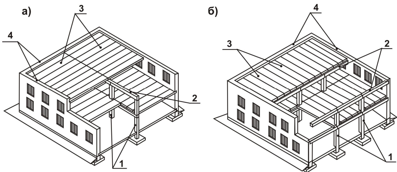
Рис. 17. Неполный каркас
