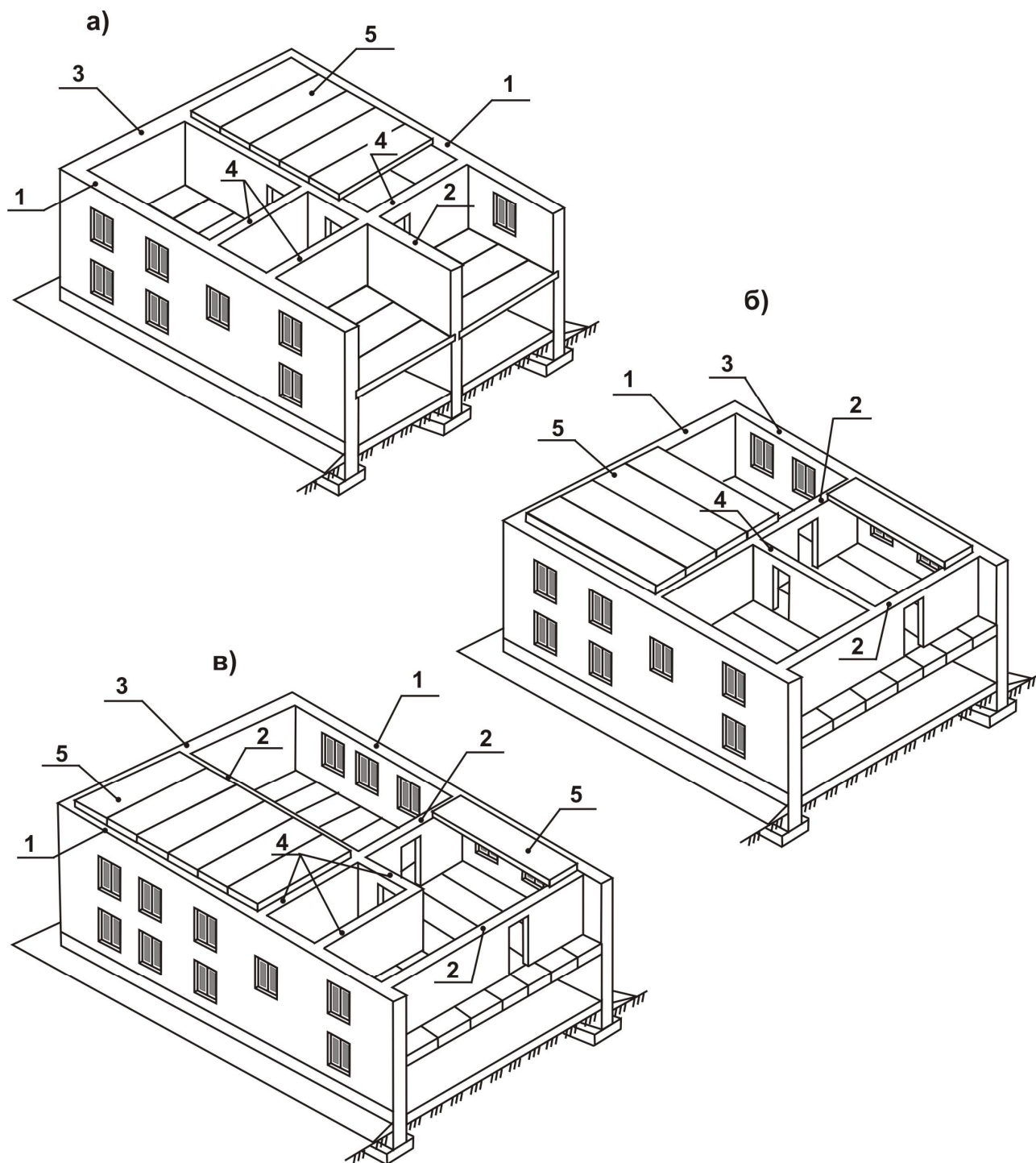
Рис. 14. Виды конструктивных схем стеной конструктивной системы
