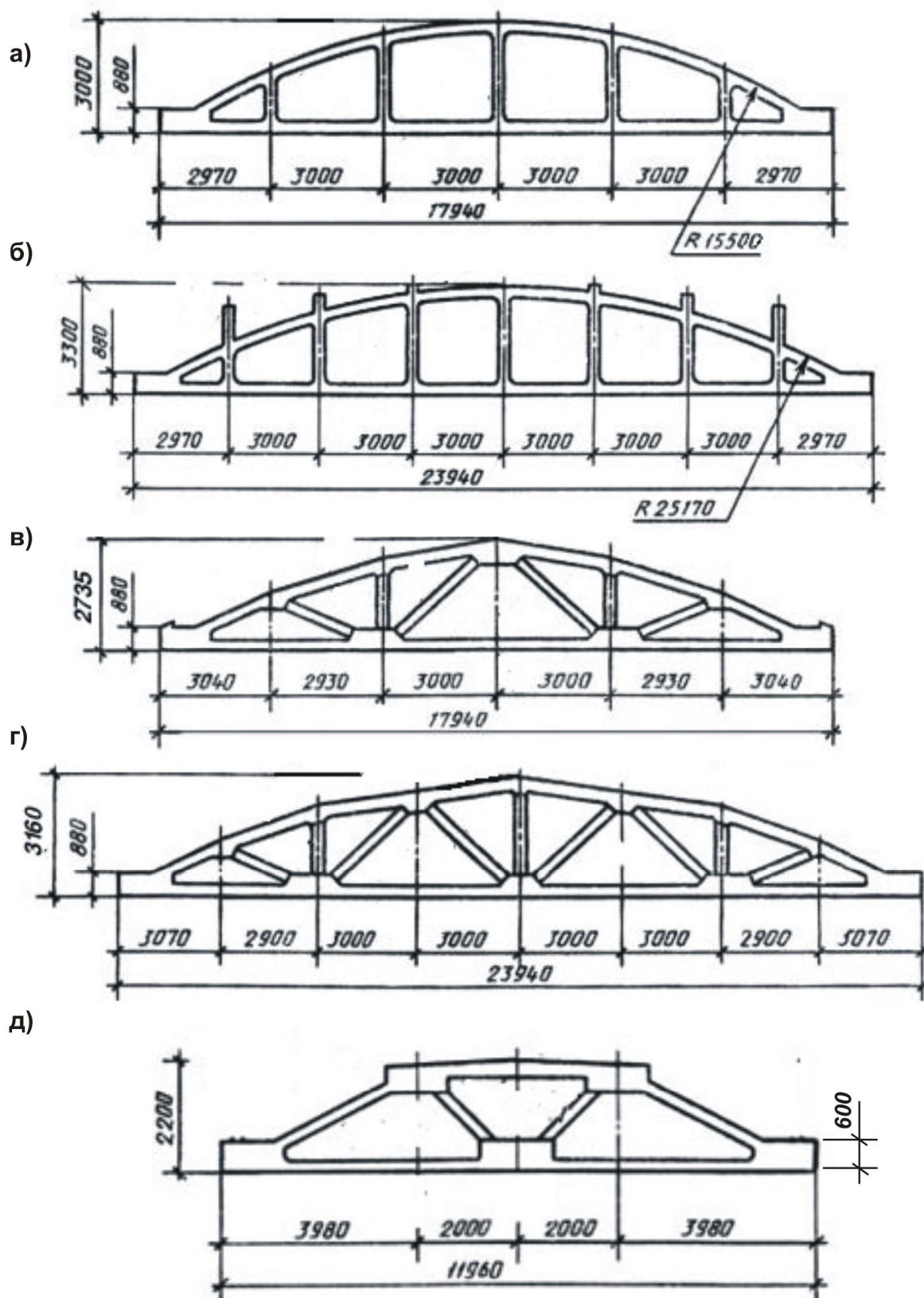
а) арочная безраскосная пролётом 18 м; б) то же, пролётом 24 м; в) сегментарная пролётом 18 м; г) то же пролётом 24 м; д) подстропильная ферма
