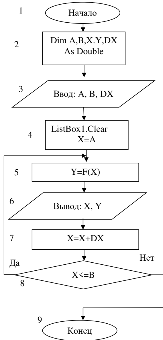
Рис. 16. Блок-схема программы Табулирование.
