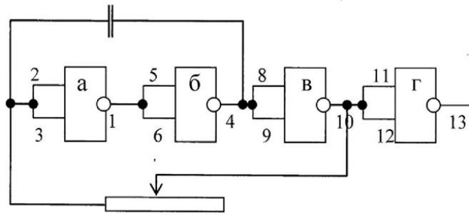
Рис.2. Принципиальная схема мультивибратора на элементах цифровой логики (микросхема к155ла8)
