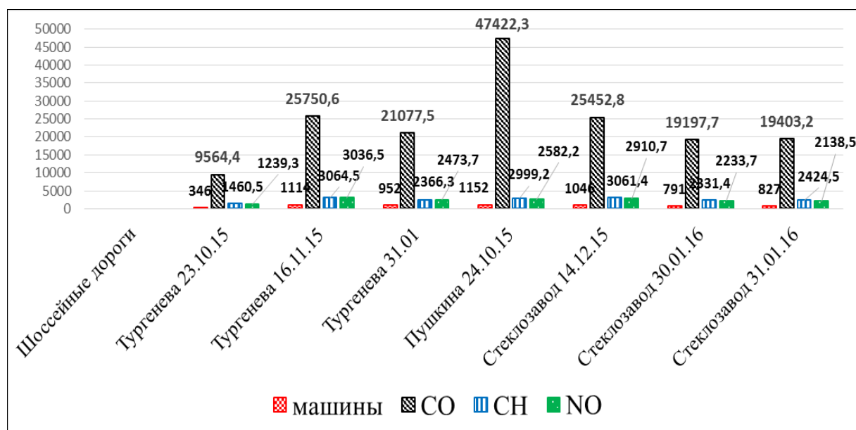
Рис. 1. Количество автомобилей и выбросов (CO, CH, NOx) на трассах г. Бор
