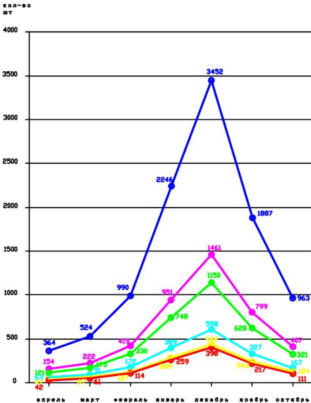
Рис 1. График потребности в трубках солнечного коллектора в зависимости от месяца: с апреля по октябрь. Условные обозначения, по тепловым нагрузкам начиная с верхней линии: 1) тепловая нагрузка на отопление всего коттеджа; 2) то же только для второго этажа; 3) то же только для третьего этажа; 4) тепловая нагрузка на горячее водоснабжение; 5) тепловая нагрузка на отопление подвала; 6) тепловая нагрузка на лестничные клетки.
