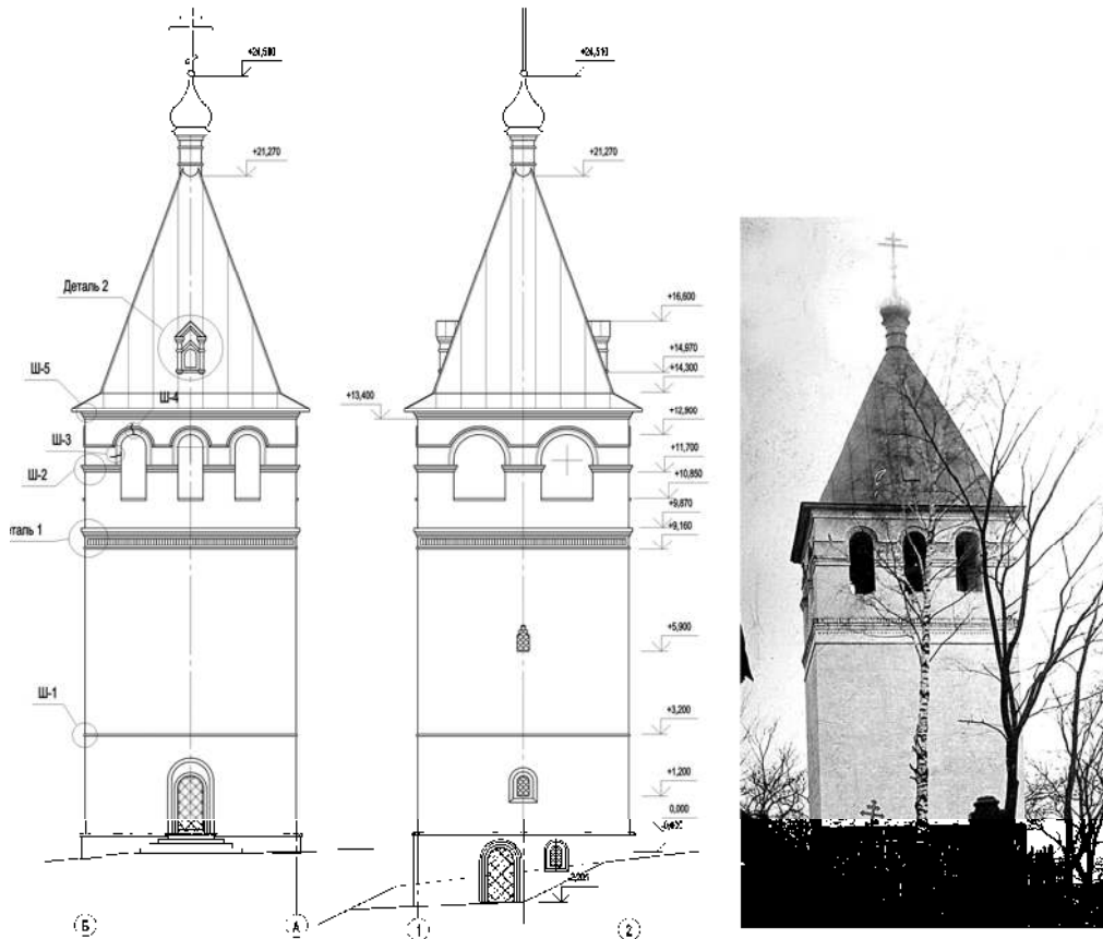
Колокольня Дудина монастыря. Фасады. Проект воссоздания. (ЗАО ТИК «Старый Нижний Новгород»). Фото XIX в. (справа).
