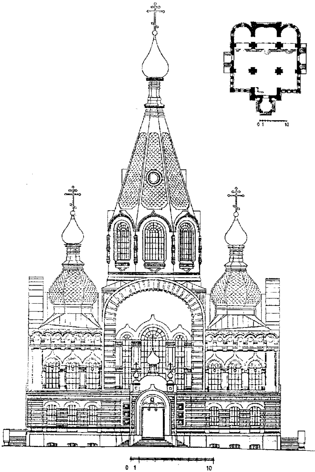
Западный фасад церкви. План 1 яруса. Проект реставрации.
