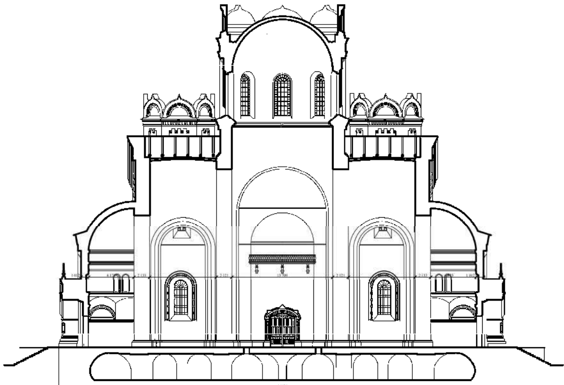
Западный фасад и разрез собора. Обмер 1984 г.
