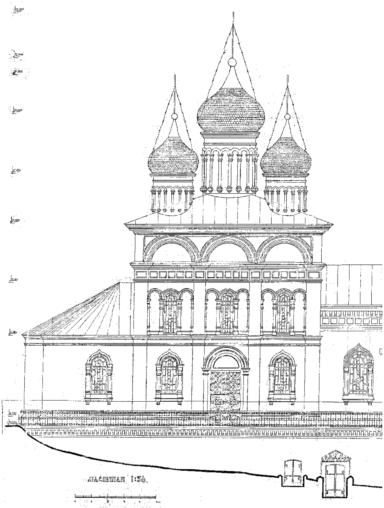
Северный фасад. Фрагмент. Проект 1993 г.
