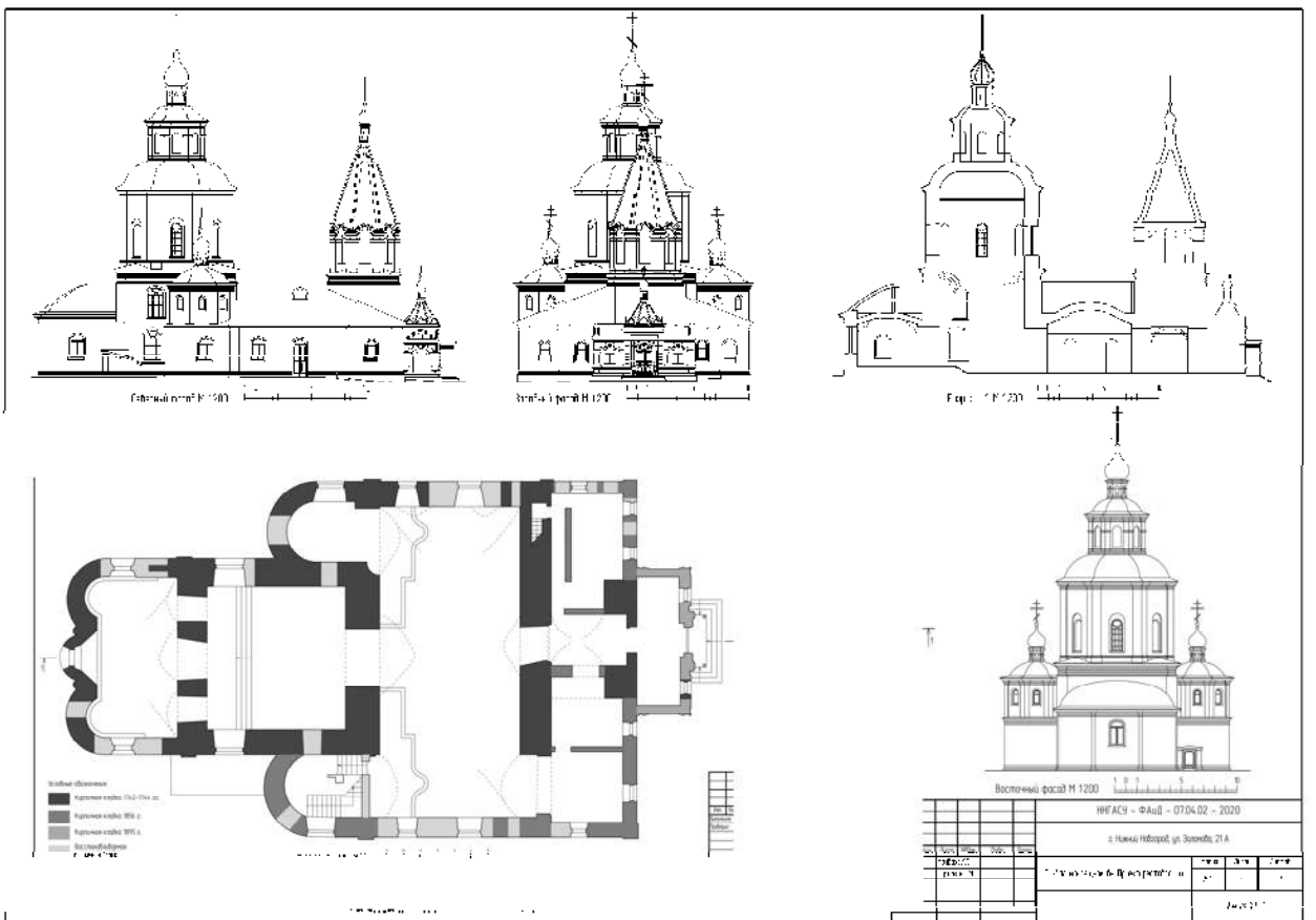
Похвалинская церковь в Нижнем Новгороде. Обмеры, проект реставрации
