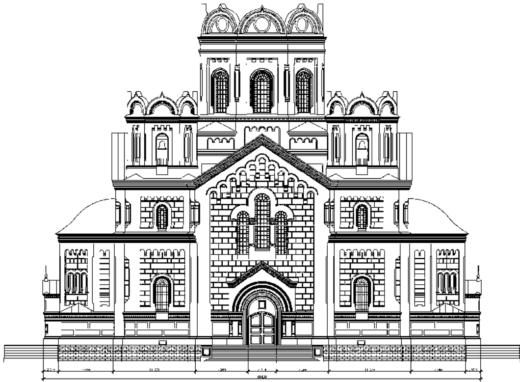
Западный фасад. Обмеры
