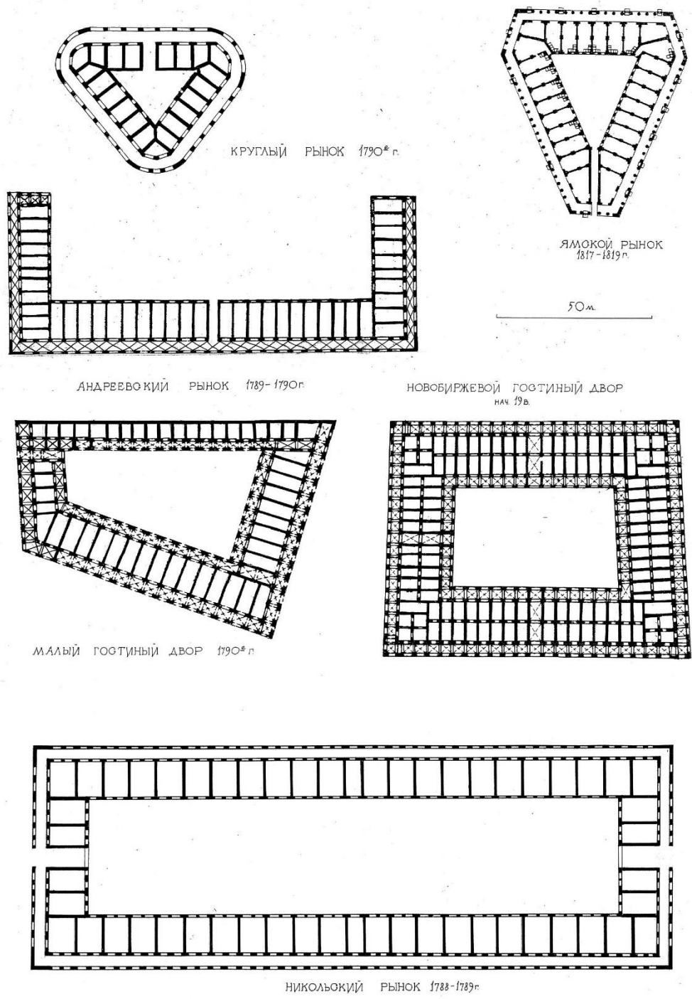
Рис. 155. Рынки Петербурга конца XVIII - начала XIX вв. Сравнение планов. Типологический ряд. Масштаб общий
