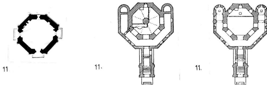
Рис. 74. Храмы с открытыми шатрами на основе разных по конфигурации четвериках. Типологический ряд
