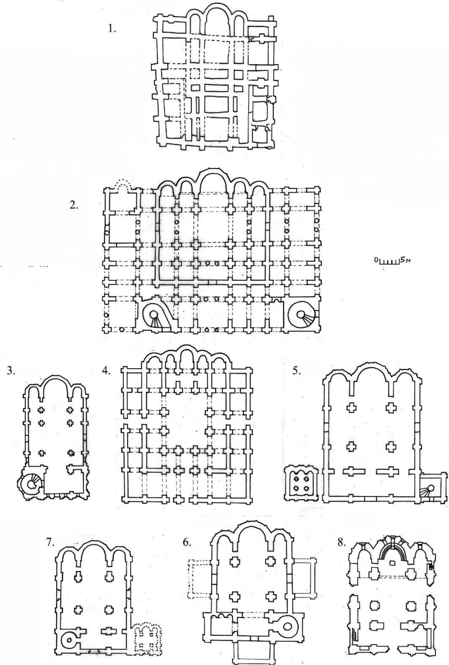
Рис. 15. Сравнение планов культовых построек Киева и окрестностей X-XII веков. Типологический ряд. Обозначения см. рис. 14
