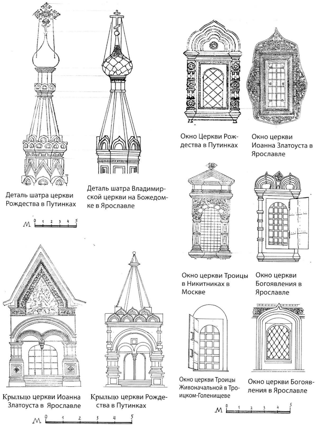
Рис. 116. Сравнение архитектурных деталей Москвы и Ярославля
