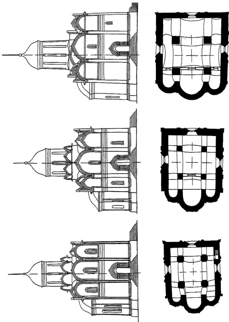
Рис. 45. Сравнение планов и фасадов соборов с рядами диагональных сводов: 1- Успенского в Звенигороде; 2- Андроникова монастыря; 3- Троице-Сергиева монастыря. Масштаб общий. Показано смещение основного входа в храм и основного барабана с куполом
