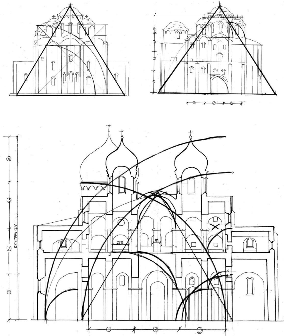
Рис. 19. Софийский собор в Новгороде. Пропорционирование построения фасадов и разреза. Использование модуля и равных соотношений длины и высоты основных элементов. Использование приема вписанных равносторонних треугольников
