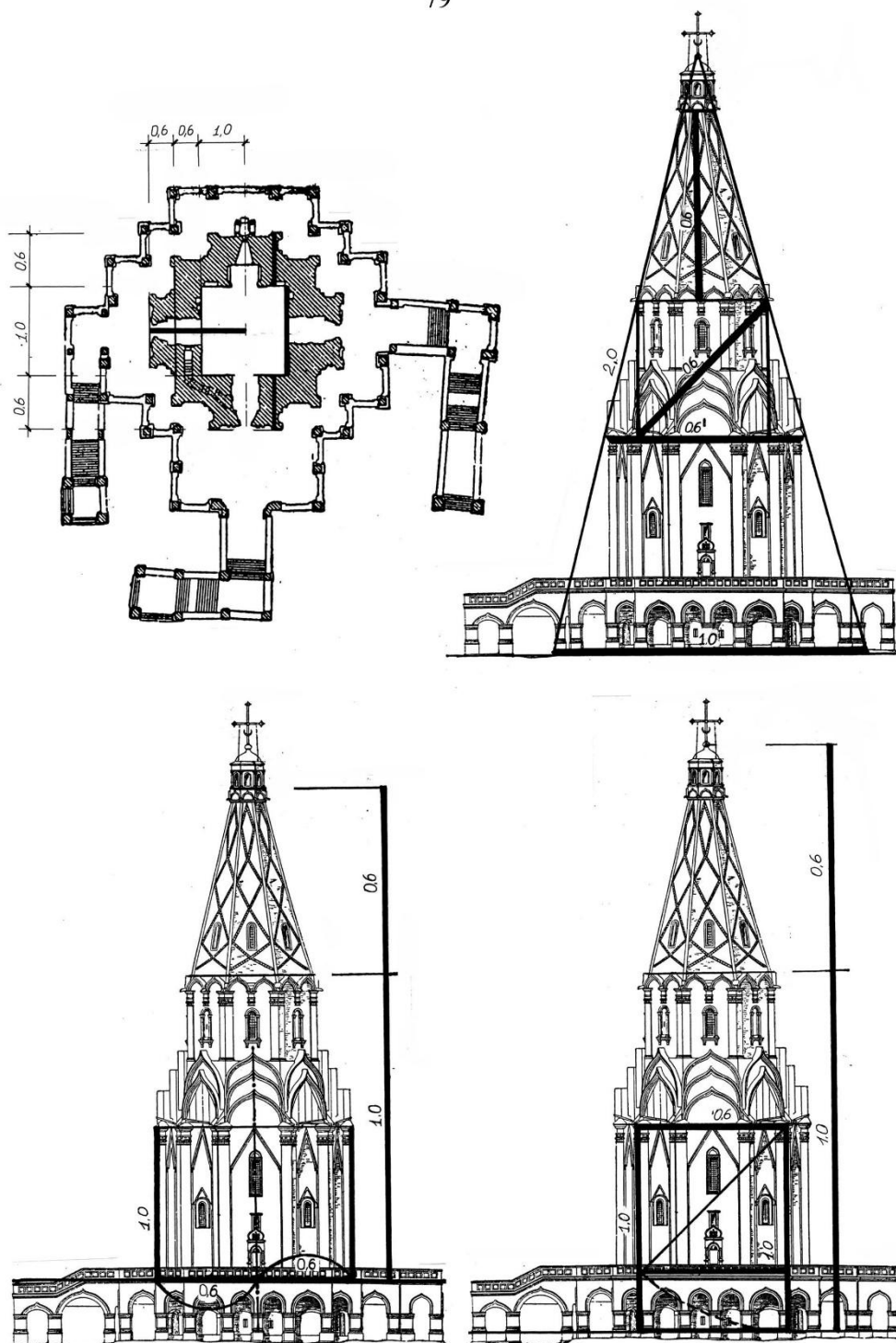
Рис. 71. Церковь Вознесения в Коломенском. Пропорциональный анализ на основе “золотого сечения” и геометрии (по Афанасьеву К.Н.)
