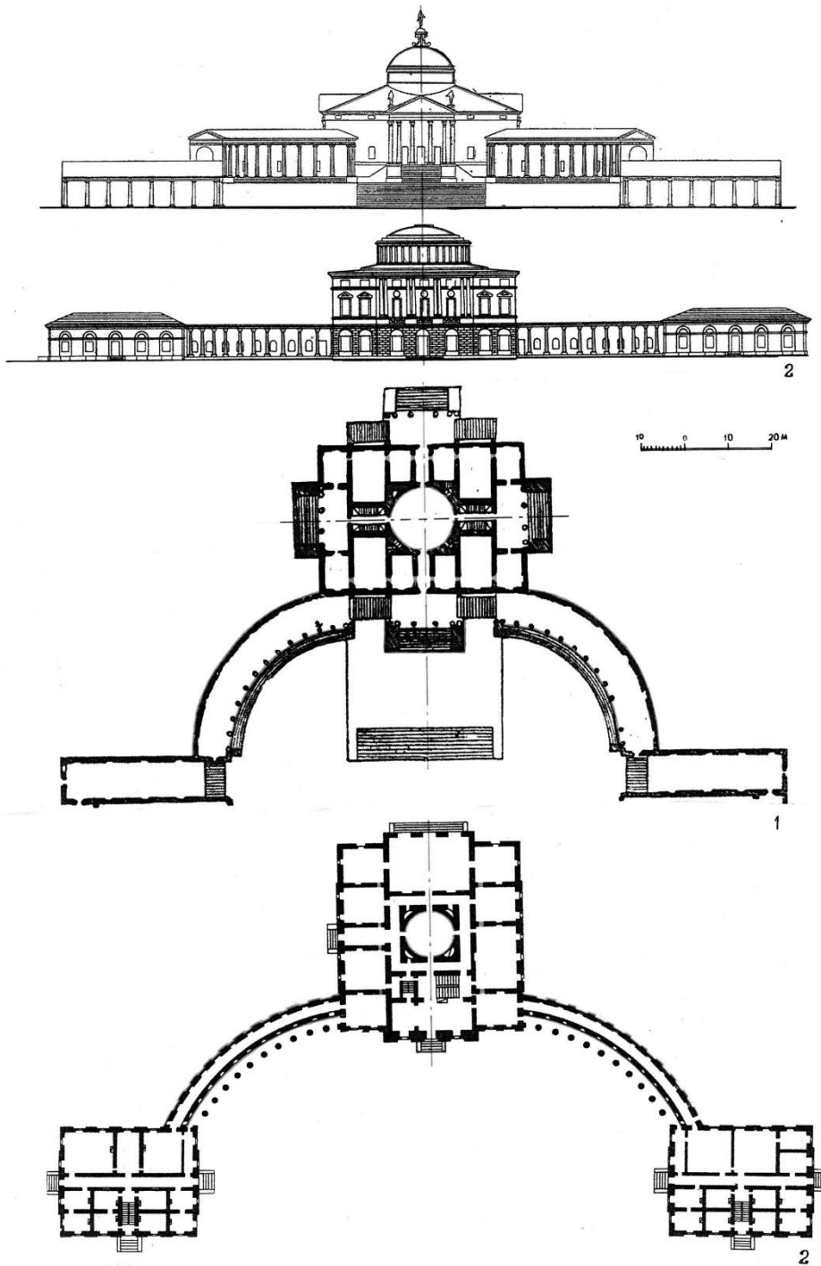
Рис. 146. Сравнение дворца в Павловске (арх. Ч. Камерон, 1786 г.) с виллой Триссино (арх. А. Палладио, 1553 г.) как образца планировки основного здания с центральным круглым залом и общего 3-частного пространственного построения. Масштаб общий
