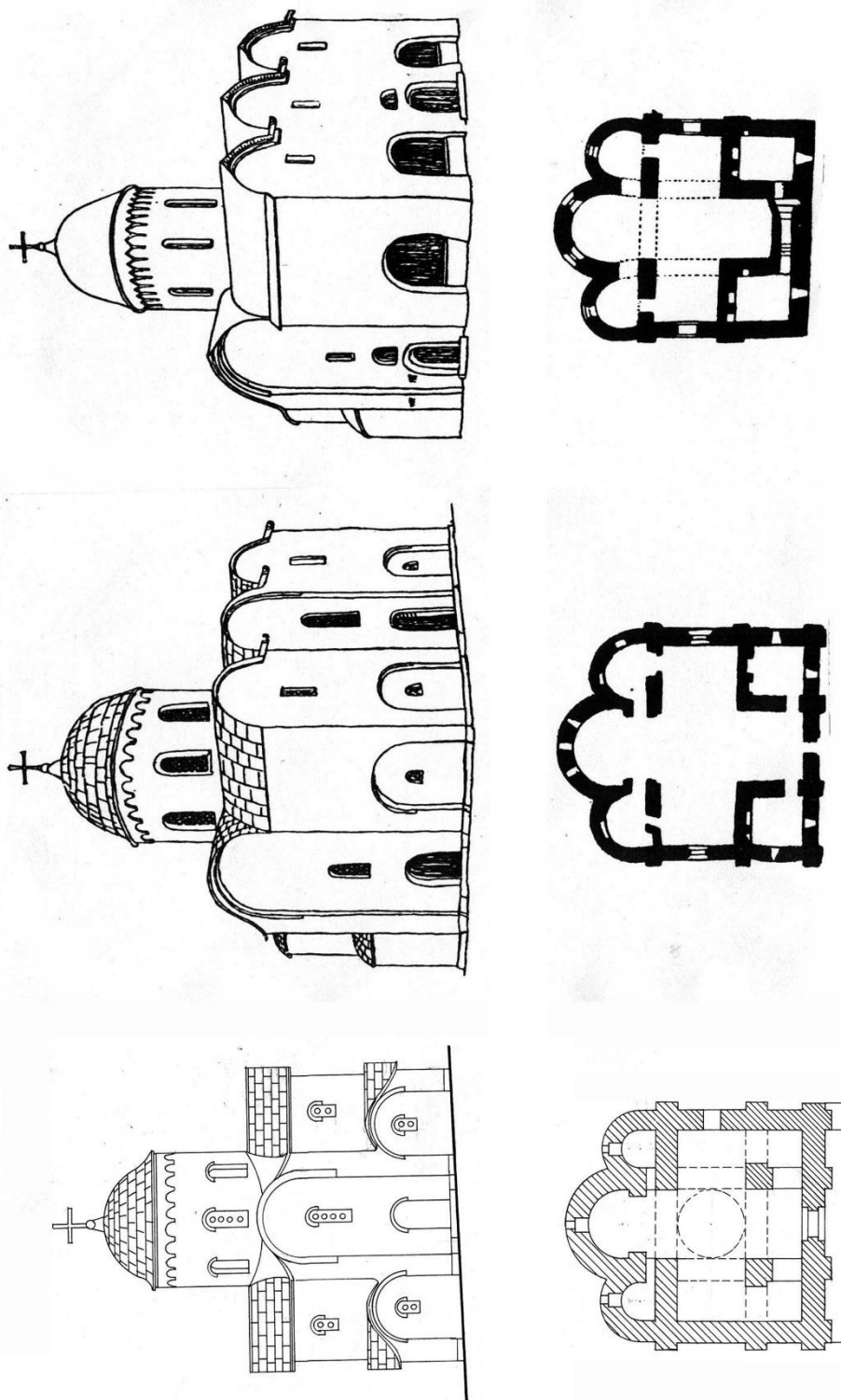
Рис. 34. Сравнение реконструкций Спасо-Преображенского собора Мирожского монастыря в Пскове (1156 г.) (вид до и после перестройки) и собора Снеготорского монастыря (1310 г.)
