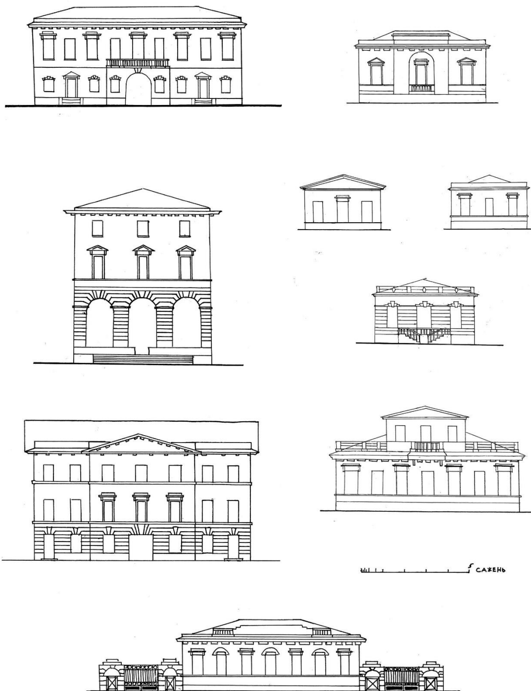
Рис. 185. Фасады образцовых проектов разных по величине жилых домов (1809 -1812 гг.). Типологический ряд. Масштаб общий
