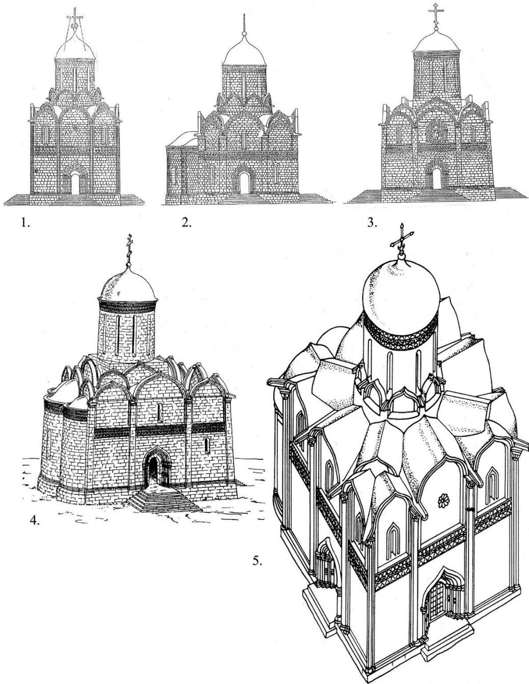
Рис. 50. Диагональные своды и кокошники в построении завершенных храмов: 1,5 - Успенского собора в Звенигороде; 2 - собора Саввино-Сторожевского монастыря; 3,4 - собора Троице-Сергиева монастыря
