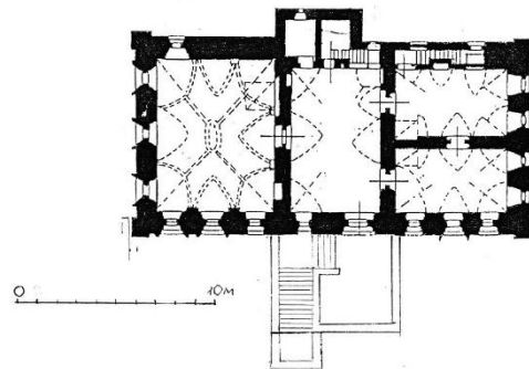
Рис. 123. Каменные дома (однопалатные и трехпалатные) в Гороховце: 1- дом Белого, 2- дом Судоплатова-Ершова, 3- дом Сапожникова-Ершова. Реконструкция
