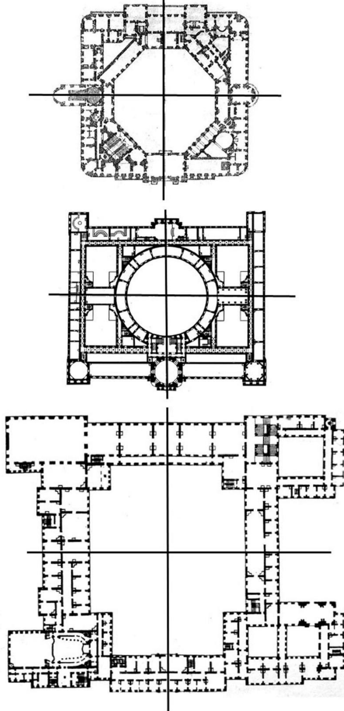
Рис. 159. Сравнение планировок крупных общественных зданий с внутренними парадными дворами: Михайловский замок, 1801 г. (вверху); Академия художеств, 1788 г. (в центре); Зимний дворец, 1762 г. (внизу). Масштаб общий
