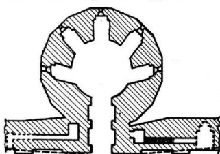
Башня Долгичевская. Планы нижнего и верхнего ярусов
