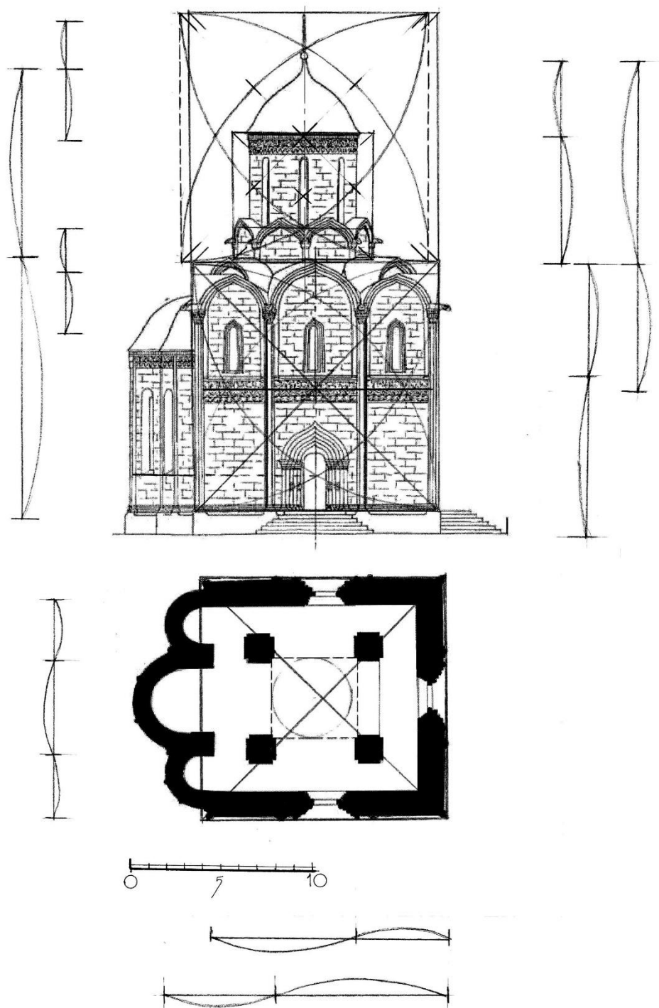
Рис. 46. Успенский собор в Звенигороде. Показаны пропорциональные ряды на основе "золотого сечения" в построении основных объемов храма и основных членений
