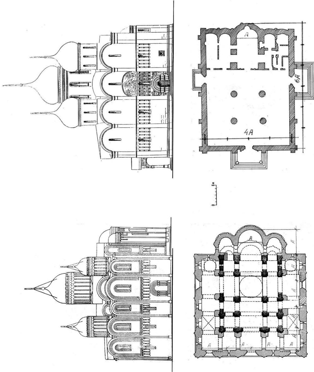
Рис. 55. Сравнение фасадов и планов Успенского собора во Владимире (слева) и Успенского собора Московского кремля (справа). Масштаб общий
