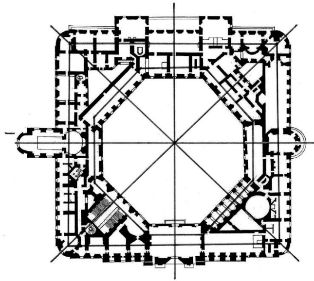
Анализ планировки залов Михайловского замка
