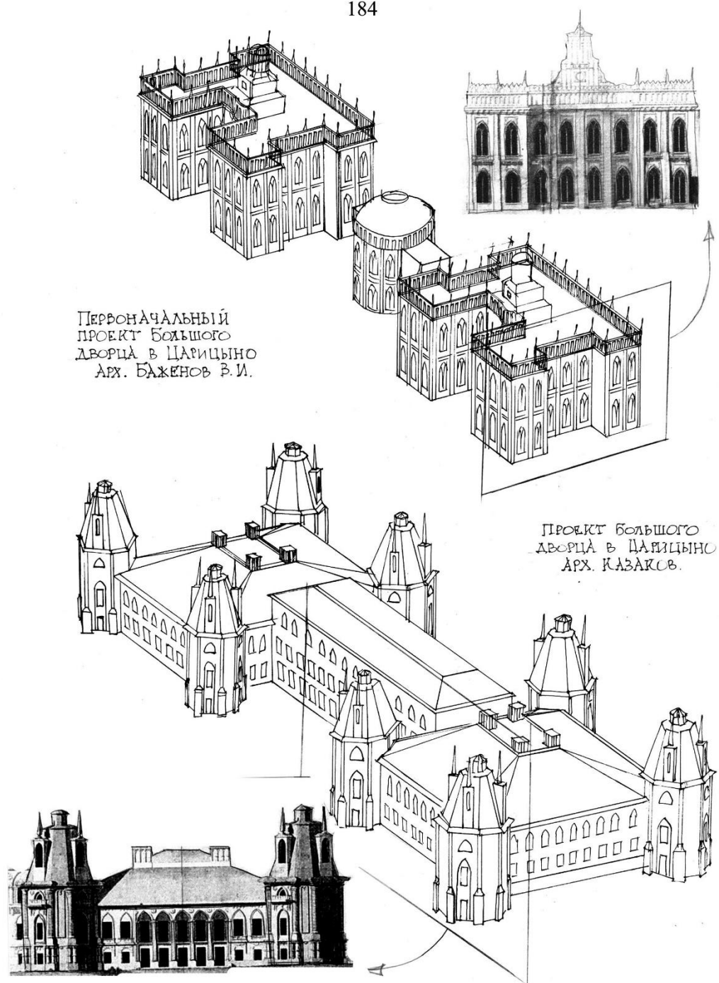
Рис. 173. Дворец в усадьбе Царицыно. Сравнение фасадов и объемной композиции дворцов по проекту арх. В.И. Баженова (вверху) и арх. М.Ф. Казакова (внизу)
