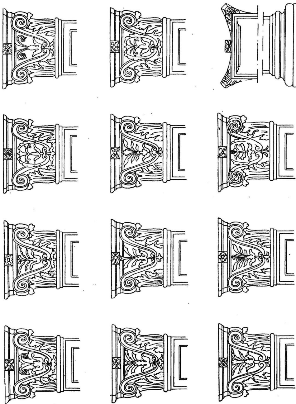
Рис. 58. Капители Архангельского собора Московского кремля. Типологический ряд, разнообразие рисунков капителей при общих габаритных размерах (по А.И. Власюку)
