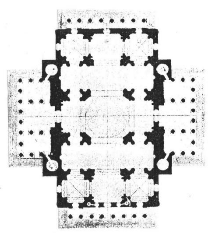
Рис. 187. Сравнение фасадов и планов Исаакиевского собора в Петербурге по проектам арх. О. Монферана, 1818 г., 1825 г., 1835 г.
