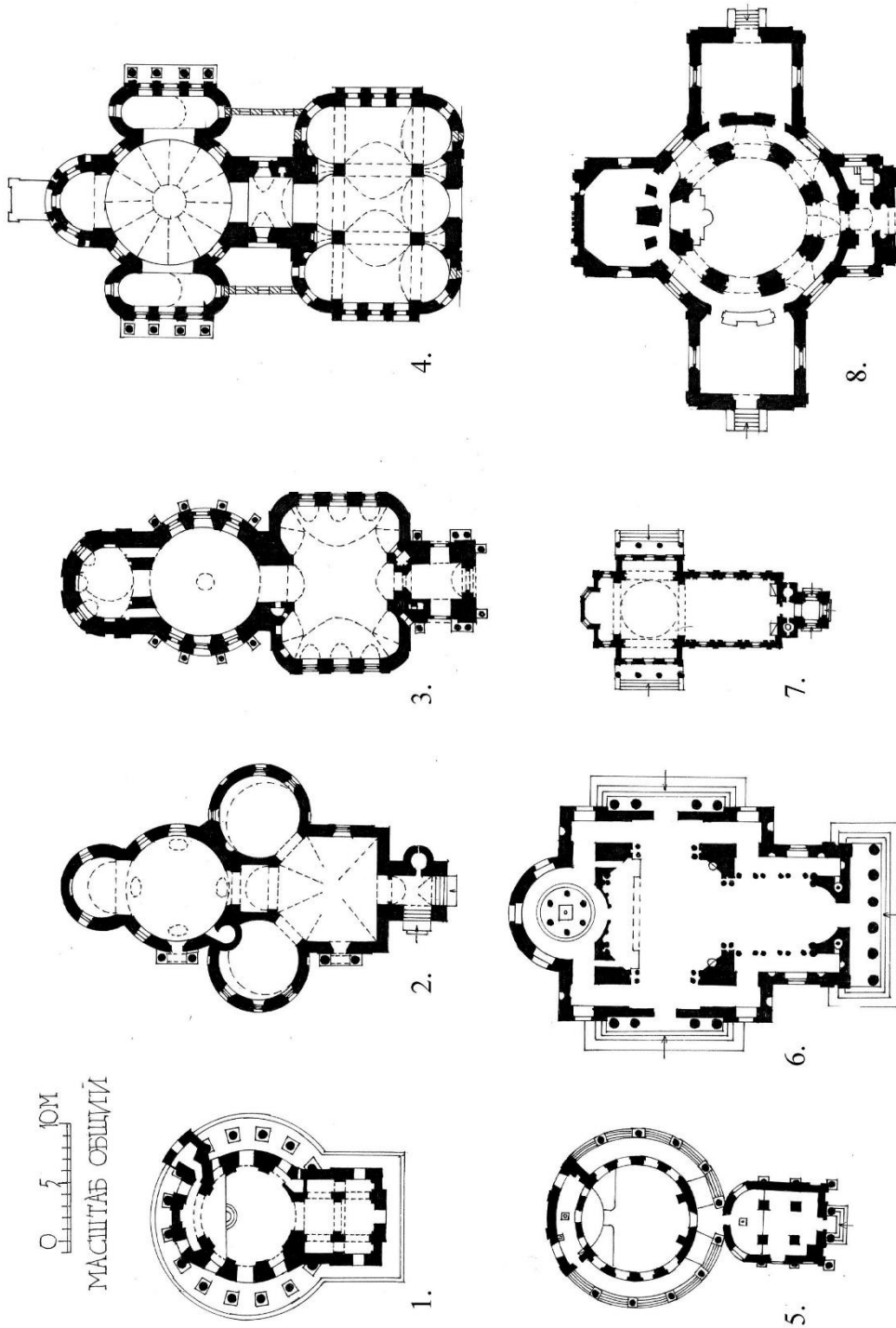
Рис. 170. Разнообразие планов церквей-ротонд: ротондальный храм (1-5,8) и храм с завершением в виде ротонды (6,7). Типологический ряд. Масштаб общий
