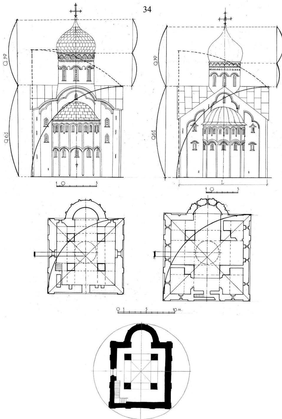
Рис. 28. Церковь Федора Стратилата (слева) и церковь Спаса Преображения (справа). Пропорционирование восточных фасадов, приведенных к одной ширине, на основе золотого сечения. На планах показано смещение центра купола относительно центральной оси объема храма
