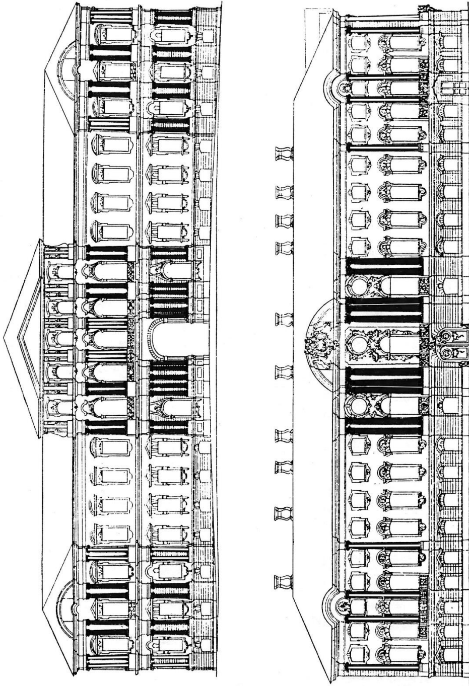
Рис. 135. Сравнение фасадов дворцов Строганова и Воронцова в Петербурге. Показано 3-частное деление фасада и использование в пластике стен колонн (заливка тоном) и пилястр (жирная линия)
