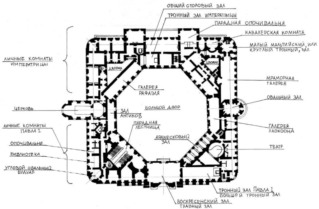
Рис. 160. Михайловский замок в Петербурге. Анализ планировки парадного второго этажа (вверху). Анализ назначения помещений (жилые и парадные). Выявлены парадные залы музейно-выставочного назначения
