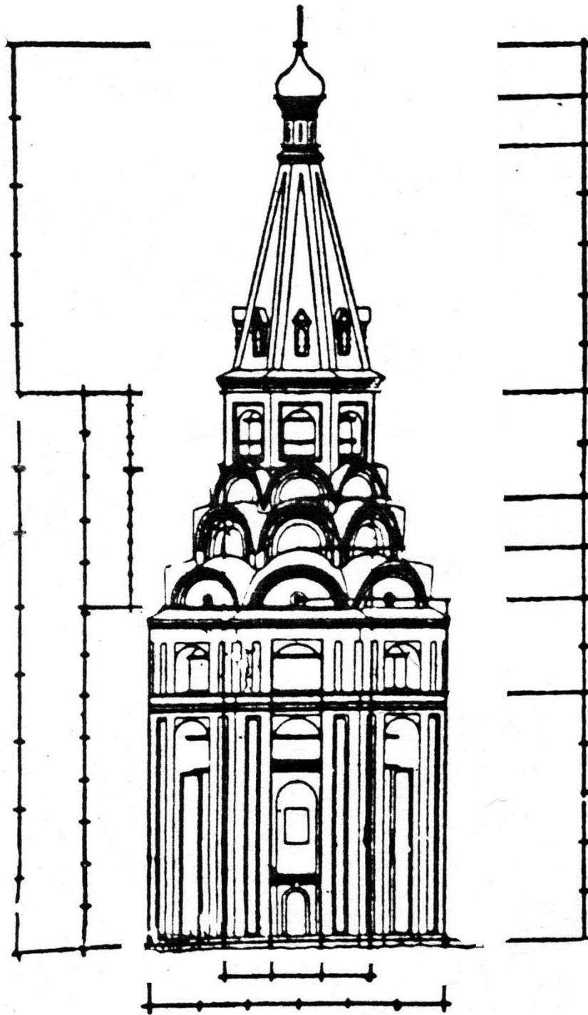
Рис. 72. Колокольня Успенского монастыря в Александрове. Пропорциональный анализ на основе "золотого сечения" с кратным соотношением 5:8 (по Максиму П.Н.)
