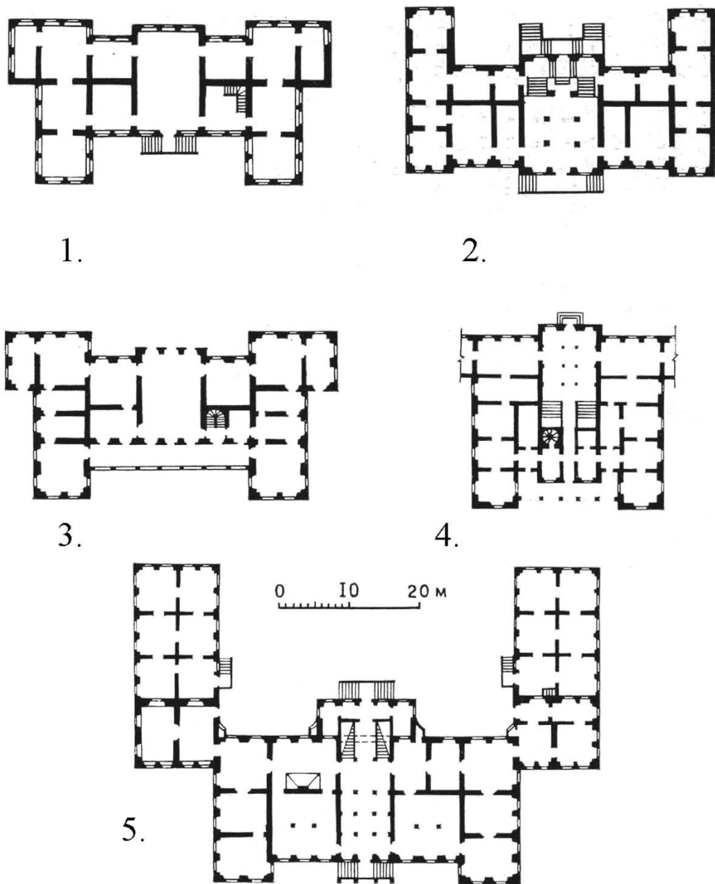
Рис. 125. Сравнение планировки дворцов Петербурга и окрестностей первой трети XVIII в. 1- палаты А.В. Кикина, 2- дом В.А. Лопухина, 3- Большой дворец в Петергофе, 4- дворец А.Д. Меншикова в Петербурге, 5- дворец А.Д. Меншикова в Ораниенбауме. (по Ю.Трубникову). Масштаб общий
