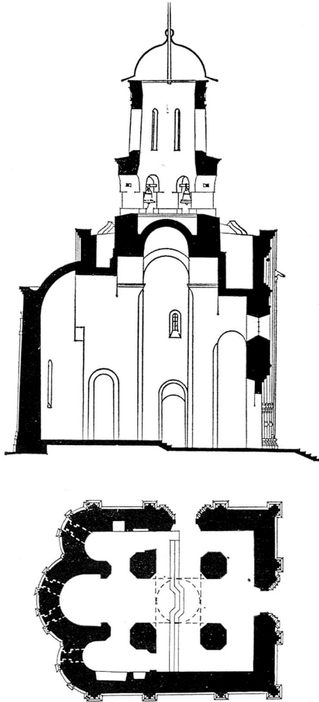
Рис. 53. Духовская церковь Троице-Сергиева монастыря, XV в. Реконструкция (по В.И. Балдину)
