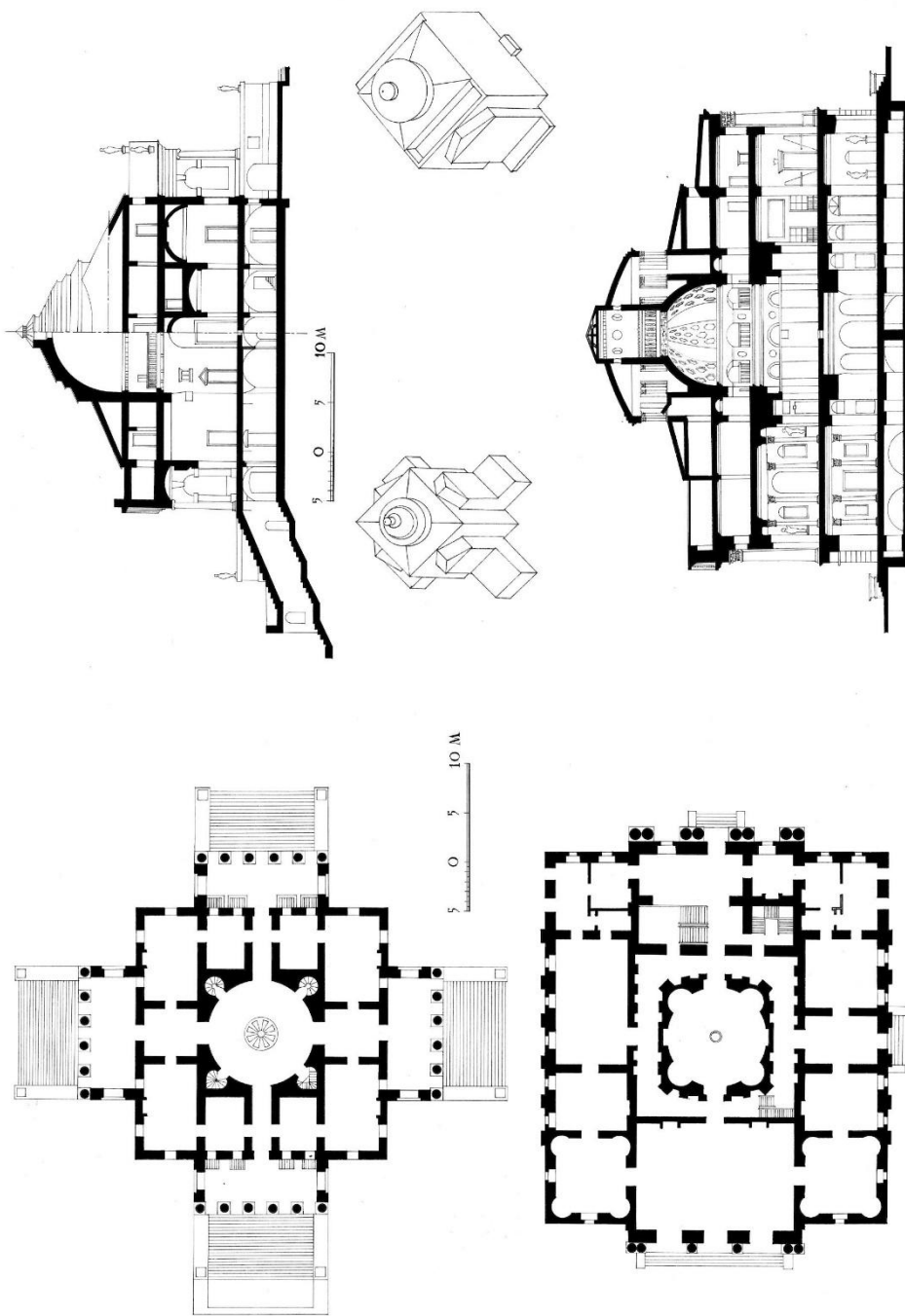
Рис. 147. Сравнение плана и разреза Павловского дворца (внизу) с виллой Альмерико - Ротонда (вверху) как прямого аналога подражания: центральный купольный зал, выявленный в симметричной объемной композиции здания. Масштаб общий
