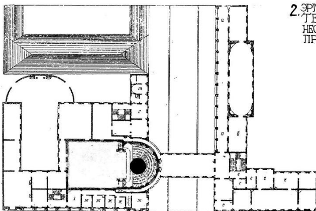
Рис. 165. Театры в планировках императорских дворцов: 1- театр Зимнего дворца, 1762 г., арх. Ф. Растрелли; 2- Эрмитажный театр, 1787 г., арх. Д. Кваренги
