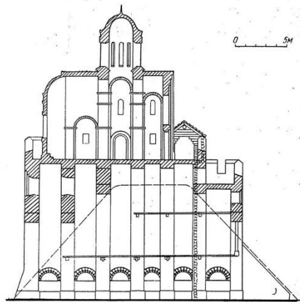
Золотые ворота в Киеве XI-XIII вв. Продольный разрез. Реконструкция С.А.Высоцкого.
