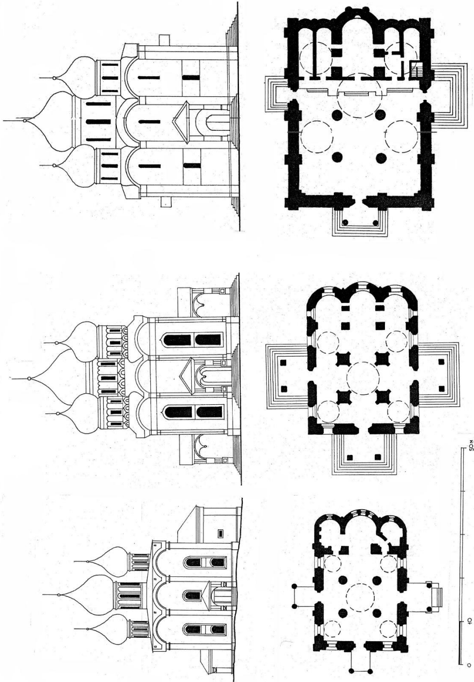
Рис. 94. Сравнение Успенского собора Московского кремля (1479 г.) (справа) с соборами XVII в.: Успенский собор монастыря Флорищева пустынь (слева), Покровский собор в Измайлово (в центре). Масштаб общий
