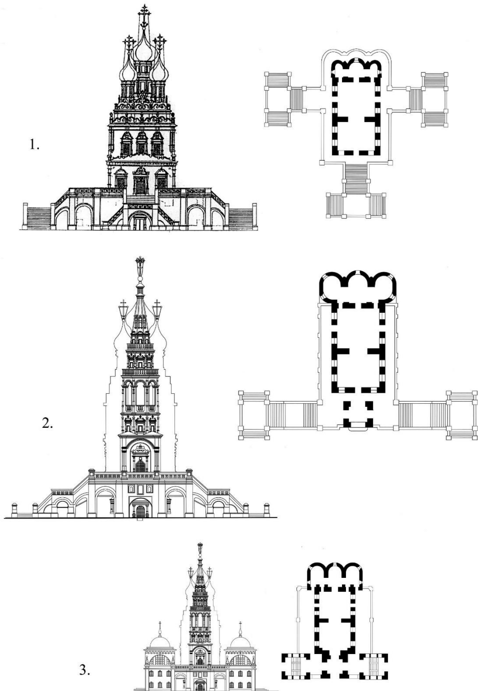
Рис. 107. Церковь Воскресения в Кадашах. Этапы строительства. Реконструкция. 1 этап - 1695 г., 2 этап - переделка крылец и постройка колокольни, 3 этап - 1802-1860 гг. - расширение входов
