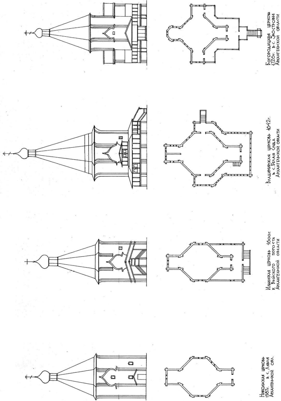
Рис. 5. Шагровые церкви восьмерикового типа. Разнообразие объемных композиций: с двумя прирубками, с прирубками и галереями, с четырьмя прирубками и галереями и крыльями, с крыльями. Масштаб общий
