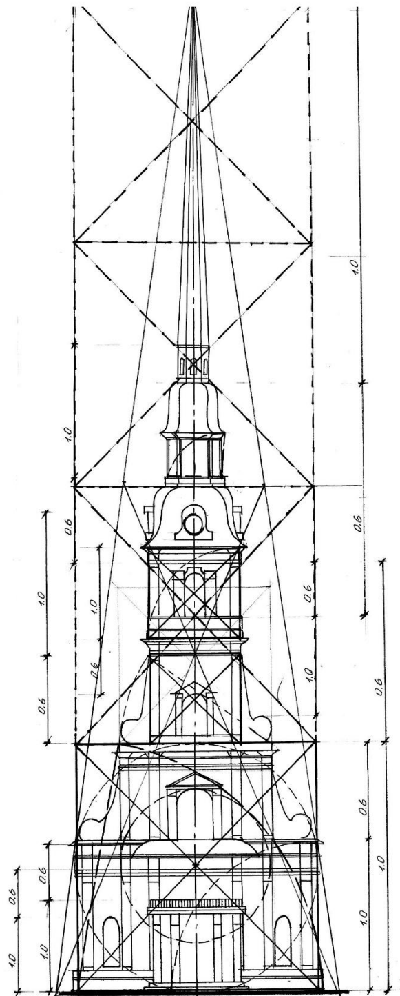
Рис. 130. Колокольня Петропавловского собора в Петербурге. Пропорциональный строй: использование модульных отношений в сочетании с “золотым сечением”
