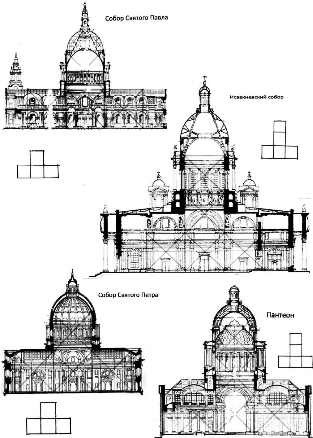
Рис. 191. Сравнение пропорционального строя разрезов с подкупольным пространством крупнейших соборов Европы
