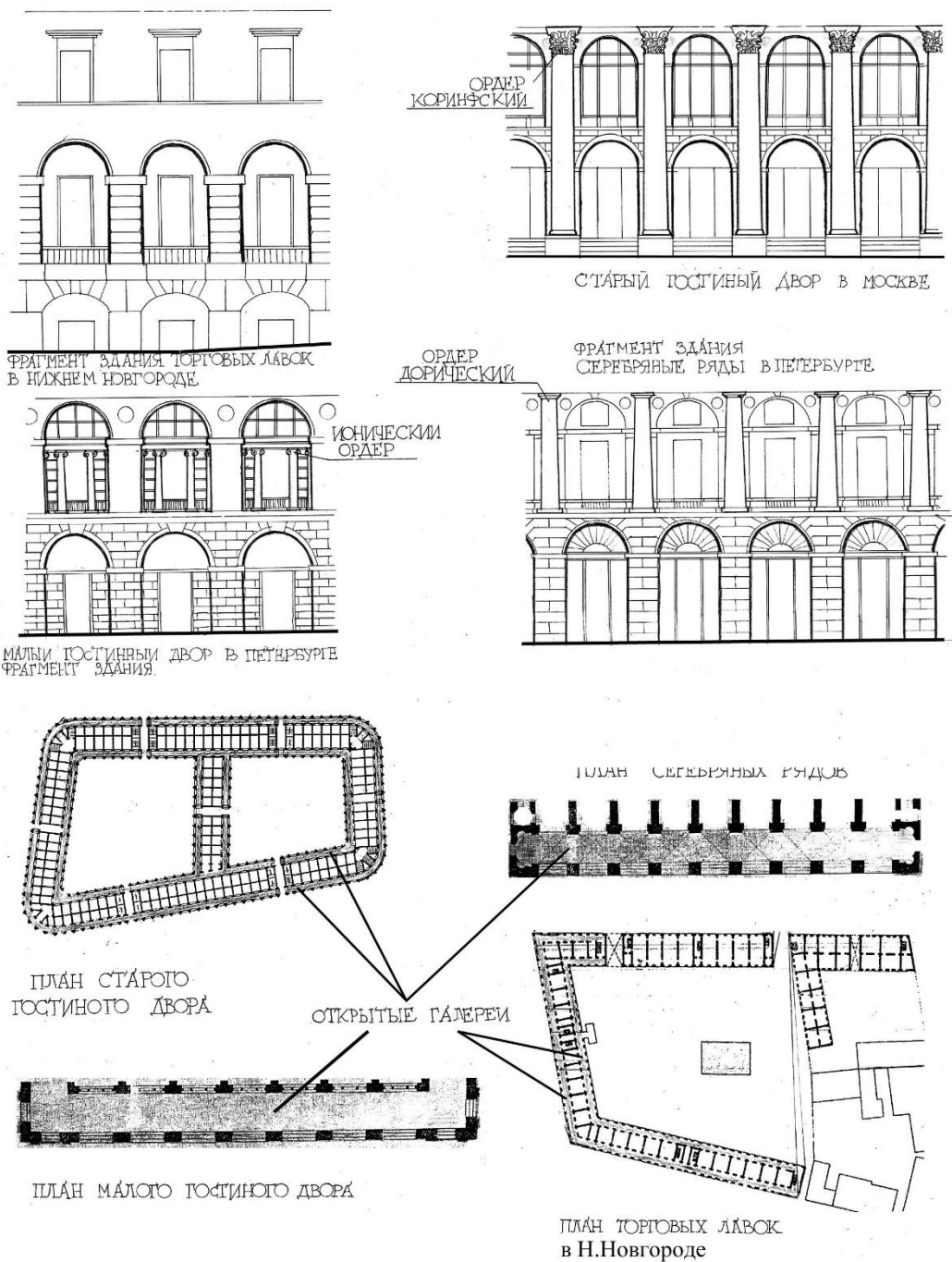
Рис. 156. Сравнение построения фасадных одно-двухъярусных ячеек открытых галерей торговых зданий Москвы, Петербурга и Н.Новгорода
