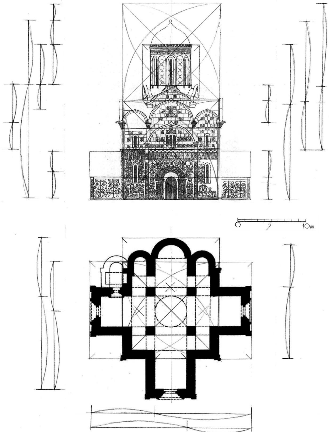
Рис. 32. Пропорционирование фасада и плана Георгиевского собора в Юрьеве - Польском на основе "золотого сечения"
