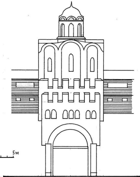
Золотые ворота в Киеве XI-XIII вв. Реконструкция С.А.Высоцкого
