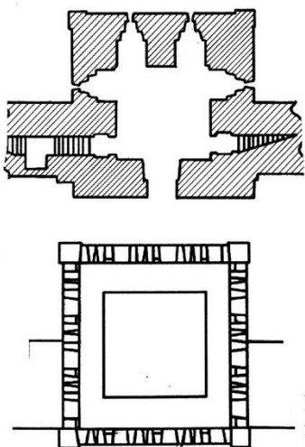
Башня Роговка: планы нижнего и верхнего ярусов
