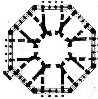
Рис. 176. Ансамбль резиденции Царицыно под Москвой. Разнообразие планировок павильонов по проектам арх. В.И. Баженова
