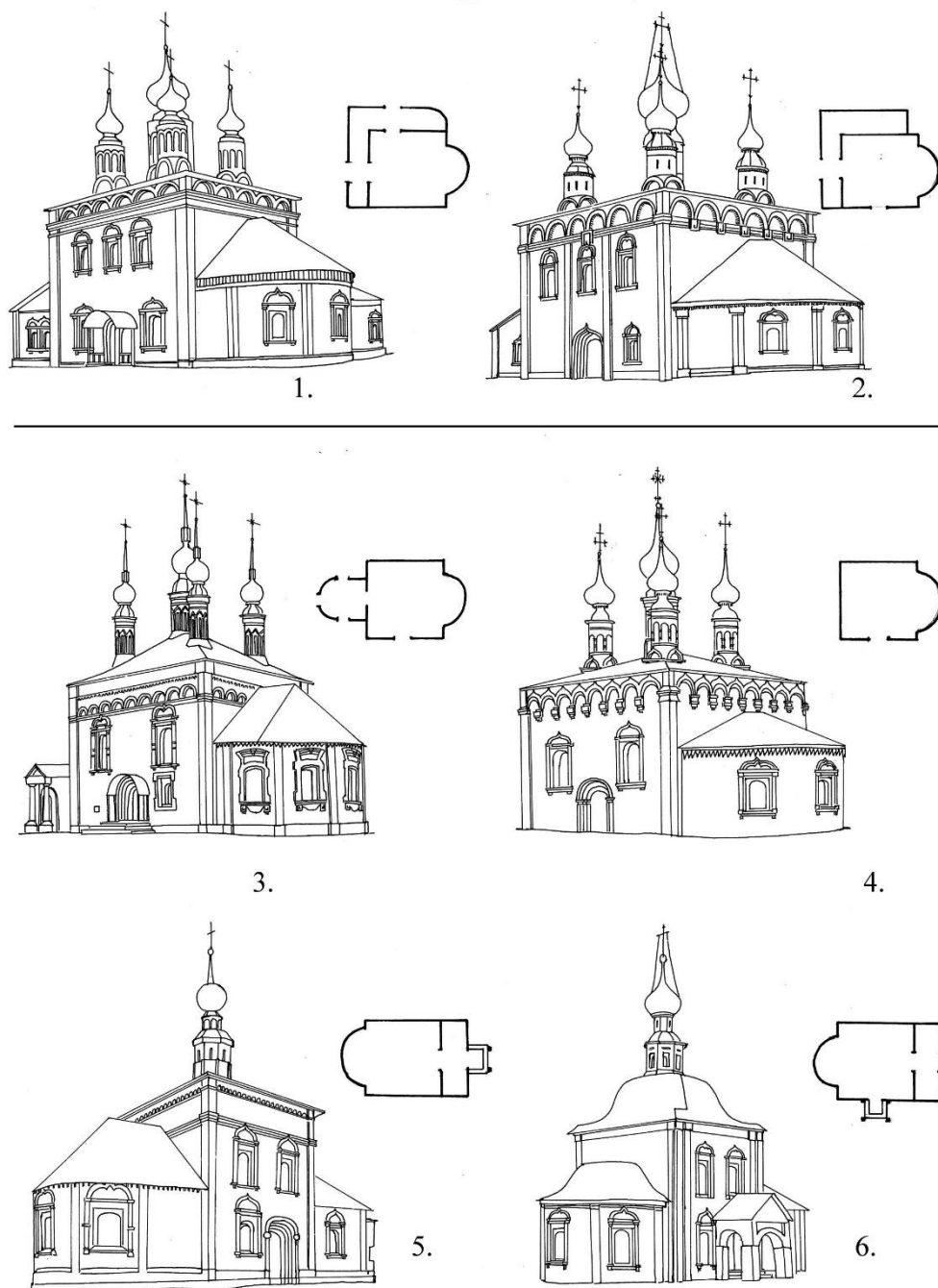
Рис. 143. Сравнение объемных композиций бесстолпных храмов в Суздале XVII-XVIII вв.: 1- Вознесенская, 1695 г., 2- Петропавловская, 1694 г., 3- Царевоконстантиновская, 1707 г., 4- Входеоерусалимская, 1707 г., 5- Знаменская, 1749 г., 6- Богоявленская, 1781 г. Проявление барокко в усилении декора фасадов, силуэта барабанов глав и покрытия
