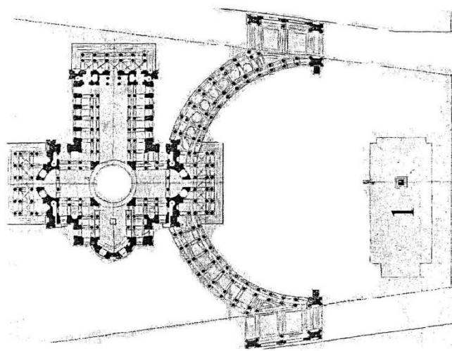
Рис. 183. Сравнение плана и разреза Казанского собора в Петербурге арх. А.Н. Воронихина и конкурсного проекта арх. Т. де Томона. Масштаб общий
