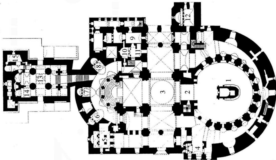
Рис. 112. Воскресенский собор Новодевичьего монастыря. Планировочное построение церкви и размещение приделов
