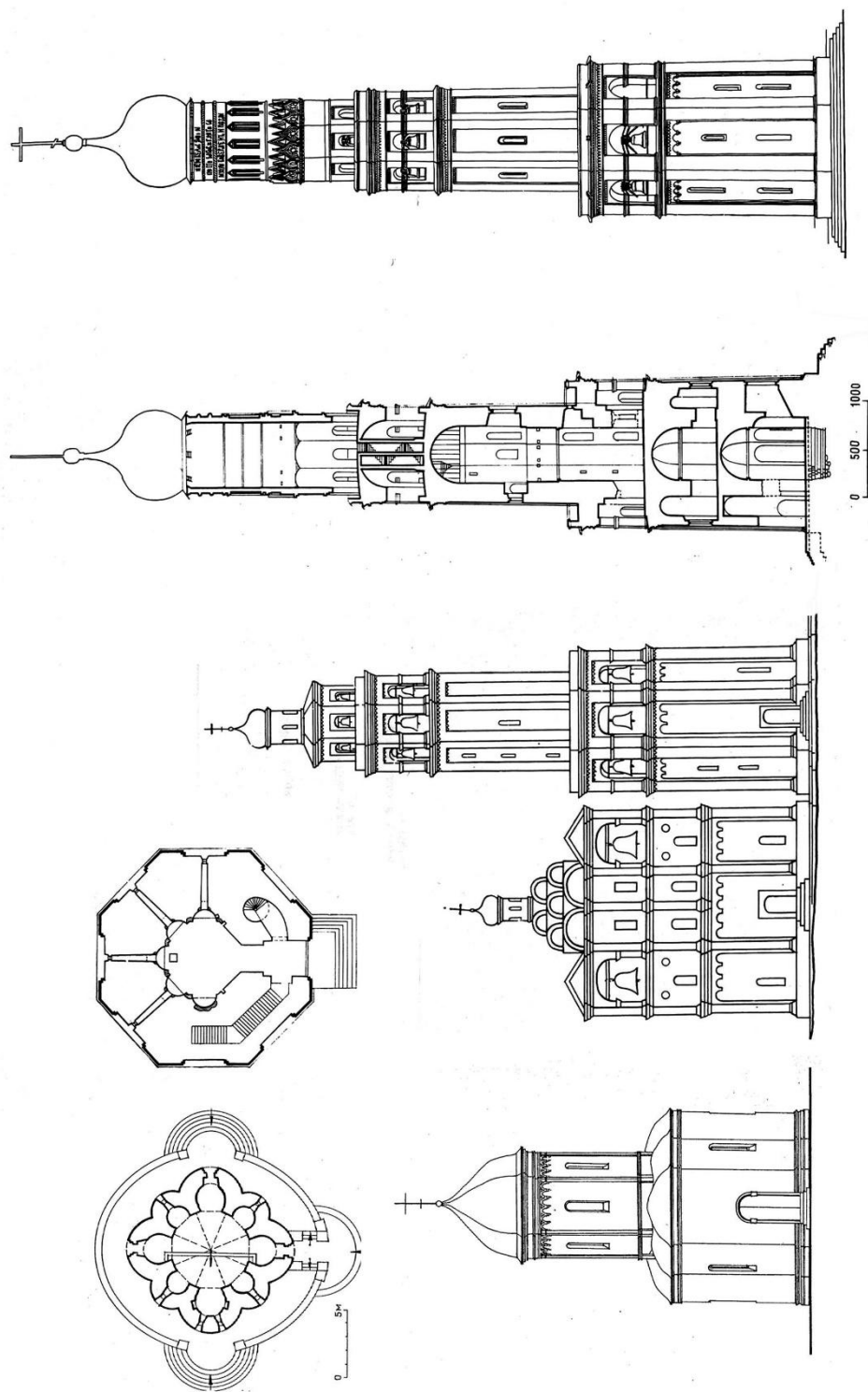
Рис. 62. Столпообразные храмы и церкви-колокольни: церковь Петра Митрополита Высоко-Петровского монастыря (слева), колокольня Ивана Великого до надстройки в начале XVI в. (в центре) и после надстройки в начале XVII в. (справа)
