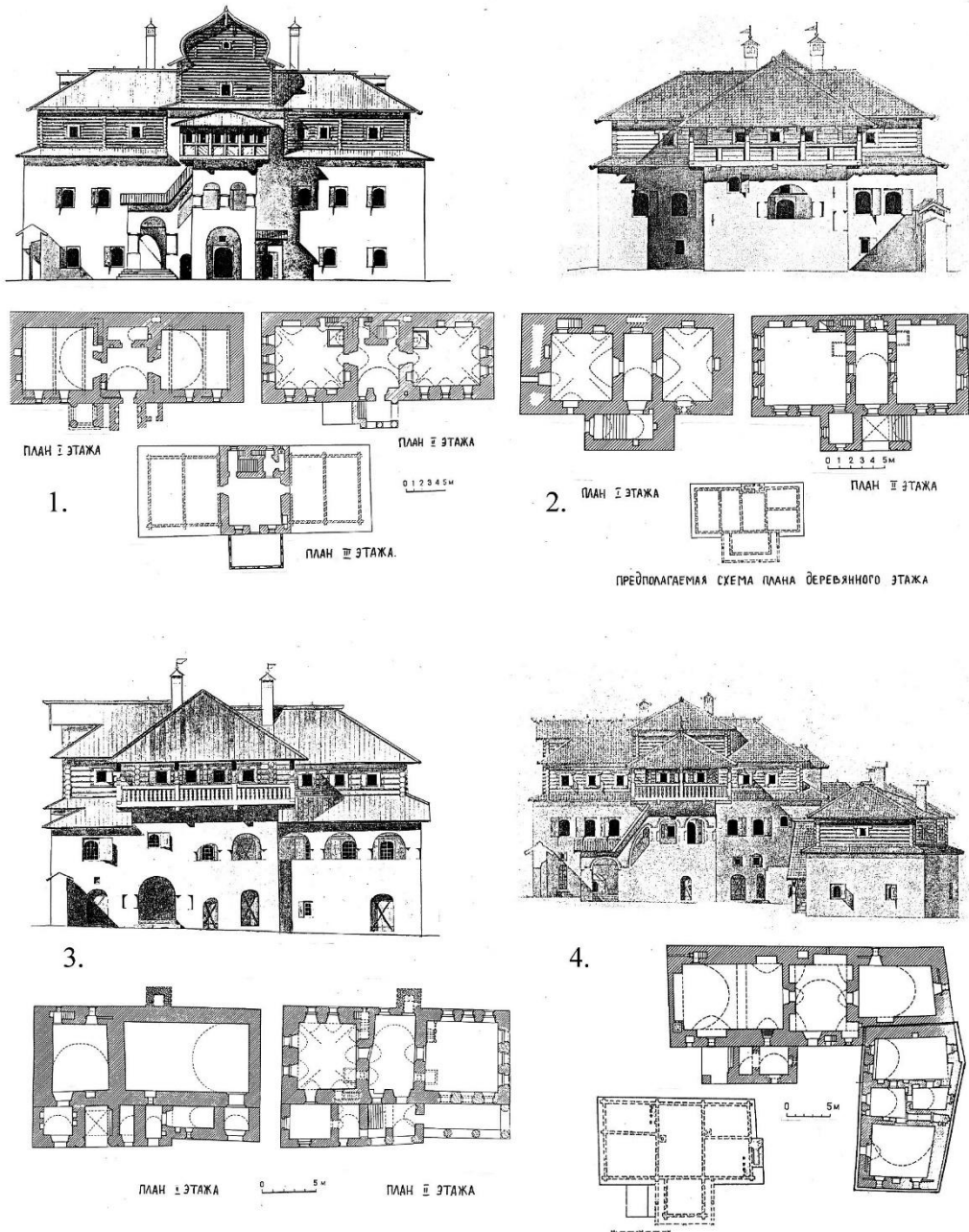
Рис. 121. Палаты Пскова с деревянными жилыми надстройками второго периода по реконструкции Ю.П. Спегальского. 1- палаты в Волчьих ямах, 2- палаты у Соколей башни, 3- палаты Ф. Гурьева, 4- дом Печенко
